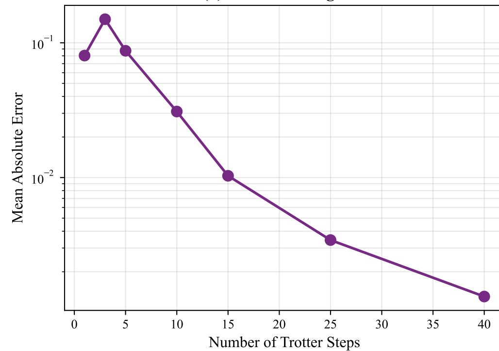
(d) Error Convergence
