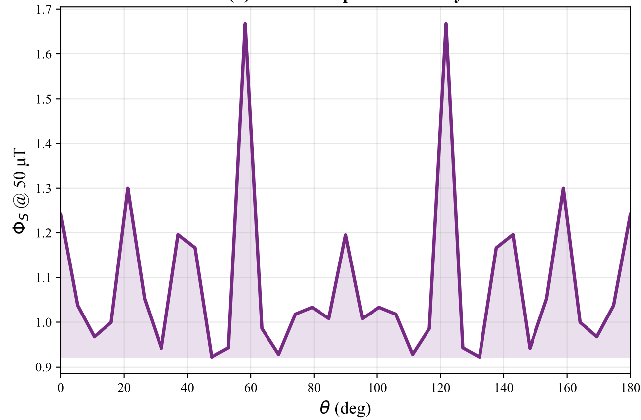
(d) Avian Compass Sensitivity
