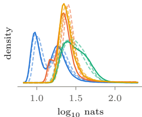
KL of \mathbf{z}
