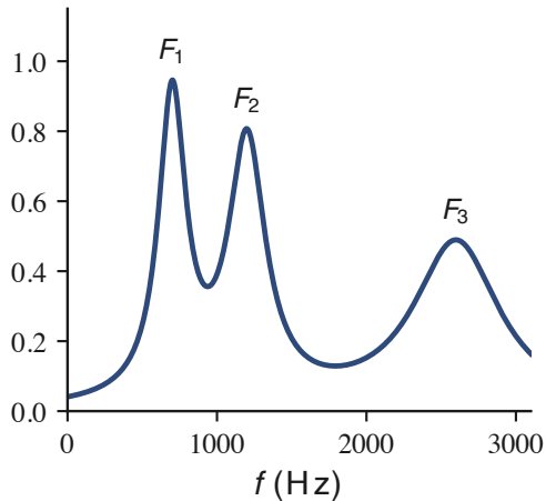
2 · filtro: tracto vocal (/a/)
