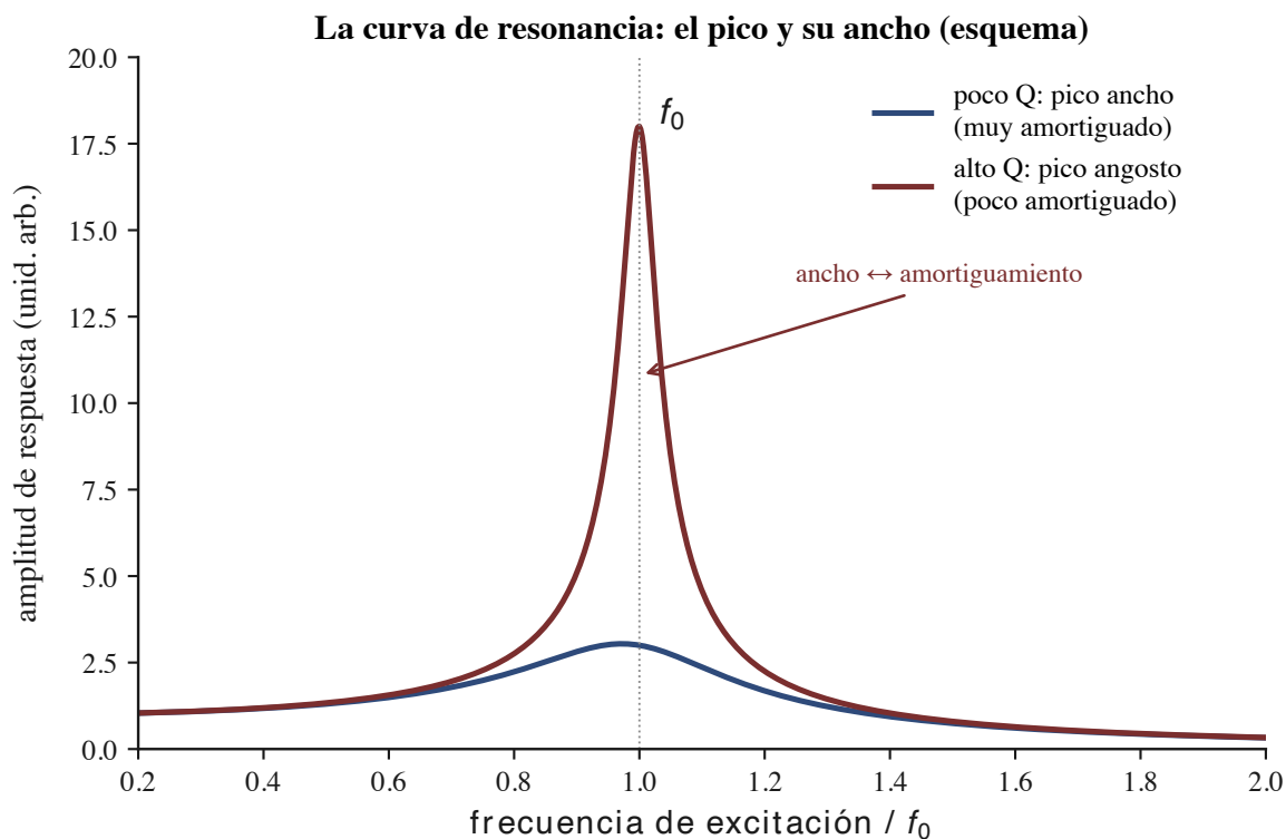
Figura 1. La curva de respuesta de un resonador (esquema): cuánto responde frente a la frecuencia con que se lo fuerza, con un pico en su frecuencia propia f_0 . Poco amortiguamiento da un pico alto y angosto (la copa de cristal, que exige su nota exacta); mucho amortiguamiento da un pico bajo y ancho (responde algo a muchas frecuencias vecinas).
