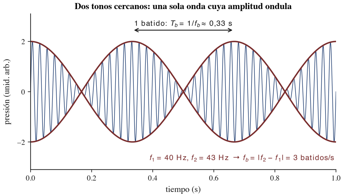
Figura 8: Figura 1. Suma de dos tonos cercanos: una onda rápida (a la frecuencia promedio) encerrada por una envolvente lenta (rojo) que sube y baja f_b = |f_2 - f_1| veces por segundo — refuerzo, silencio, refuerzo. Se dibuja con f_1 = 40 Hz y f_2 = 43 Hz para que el ciclo sea visible.
