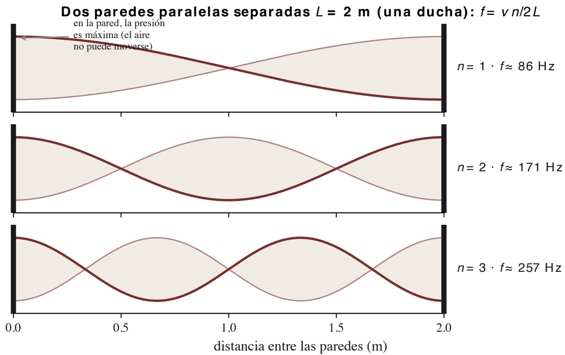
Figura 15: Figura 2. Los tres primeros modos axiales entre dos paredes separadas L = 2 m: f = v n / 2L \approx 86 , 171 y 257 Hz. En la pared rígida el aire no puede moverse y la presión es máxima — al revés que en el extremo abierto de los tubos de s12. Pocos modos, bien separados, en plena zona de la voz: por eso la ducha tiene favoritas.
