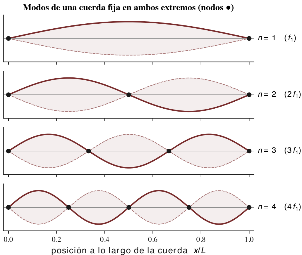
Figura 4: Figura 1. Las cuatro primeras formas de vibrar de una cuerda fija en ambos extremos: una barriga, dos, tres, cuatro. Los puntos negros (●) marcan los nodos , que no se mueven. Lo extraordinario no son las formas sino las frecuencias: el modo de n barrigas vibra a n veces la frecuencia del fundamental.
