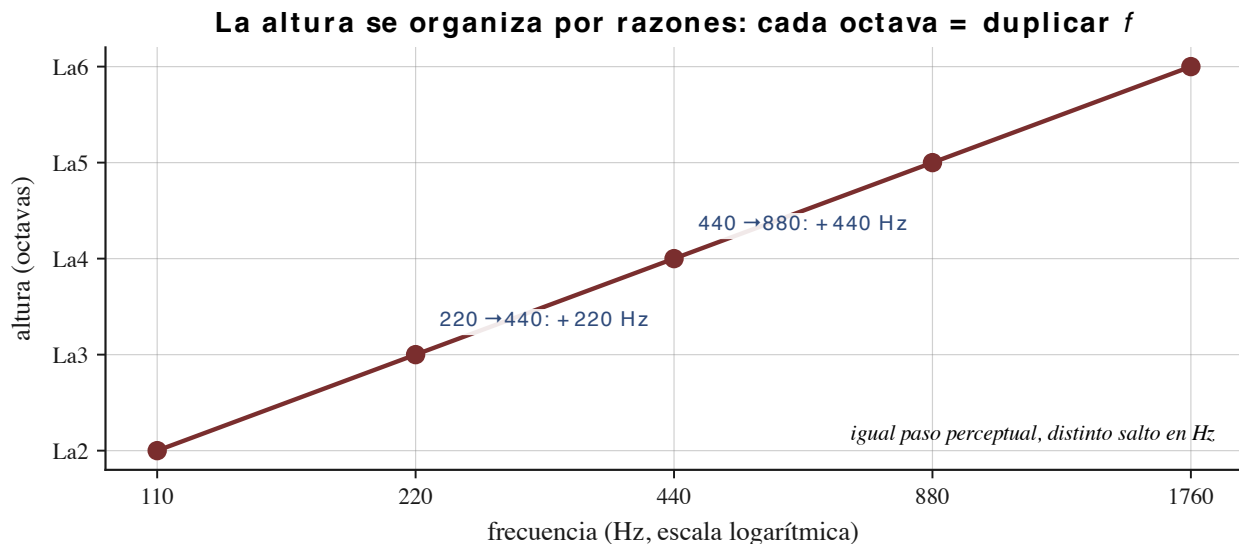
Figura 6: Figura 2. Sobre un eje de frecuencia logarítmico, los La sucesivos (110, 220, 440, 880, 1760 Hz) quedan equiespaciados: cada octava es duplicar f . El salto 220 \rightarrow 440 (+220 Hz) y el 440 \rightarrow 880 (+440 Hz) son el mismo paso perceptual —una octava— aunque abarquen distinta cantidad de hertz. La altura corre por razones, no por diferencias.
