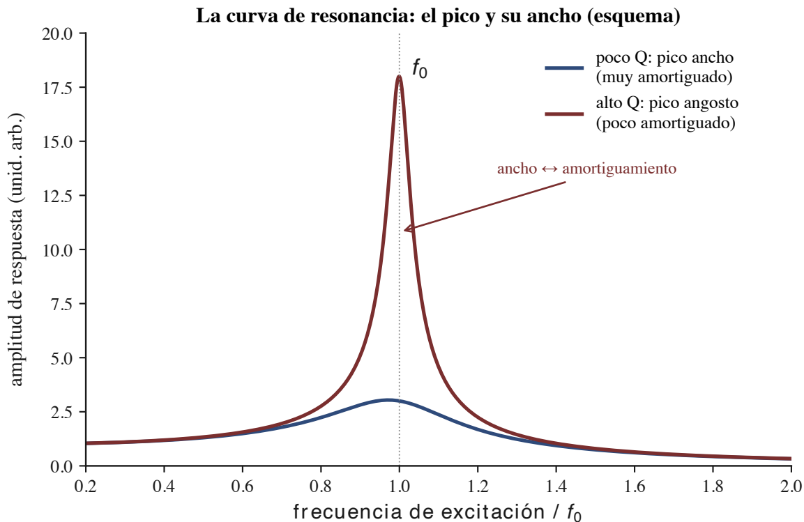
Figura 9: Figura 1. La curva de respuesta de un resonador (esquema): cuánto responde frente a la frecuencia con que se lo fuerza, con un pico en su frecuencia propia f_0 . Poco amortiguamiento da un pico alto y angosto (la copa de cristal, que exige su nota exacta); mucho amortiguamiento da un pico bajo y ancho (responde algo a muchas frecuencias vecinas).
