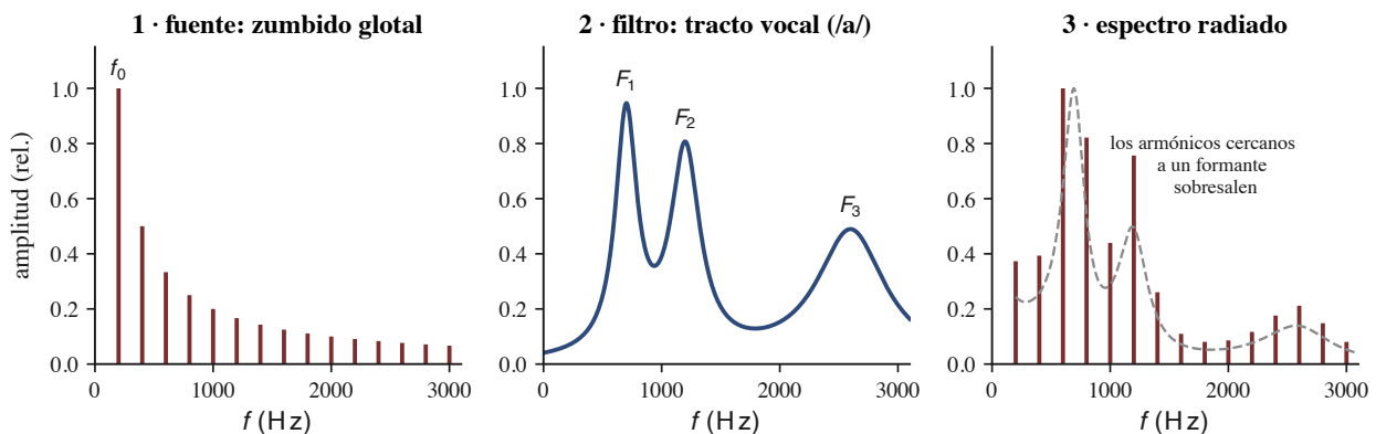
Figura 13: Figura 1. El modelo fuente-filtro en tres pasos (esquemático; una /a/ con f_0 = 200 Hz): el zumbido glotal pone el peine de armónicos, el tracto pone la envolvente de formantes, y lo radiado es el producto de ambos. La sesión hará este experimento en vivo, con su voz y el espectrograma proyectado.
