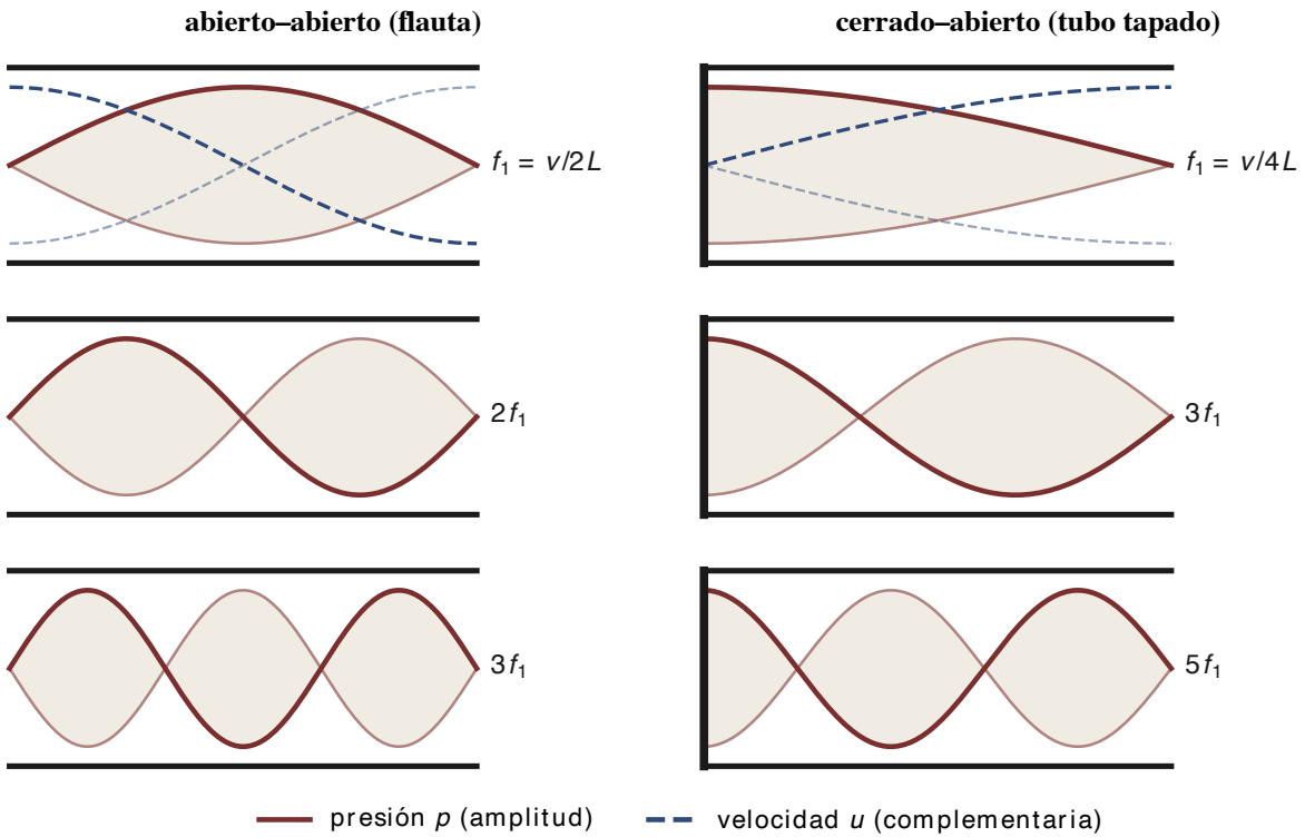
Figura 11: Figura 1. Amplitud de la onda estacionaria de presión de los tres primeros modos de un tubo abierto–abierto y de uno cerrado–abierto. La “puerta” (extremo abierto) impone un nodo de presión; la “pared” (tapa), un máximo. La velocidad del aire (punteada, primera fila) es complementaria: máxima donde la presión tiene nodo. Entre puerta y pared cabe solo un cuarto de onda: de ahí el 4L y la serie impar.
