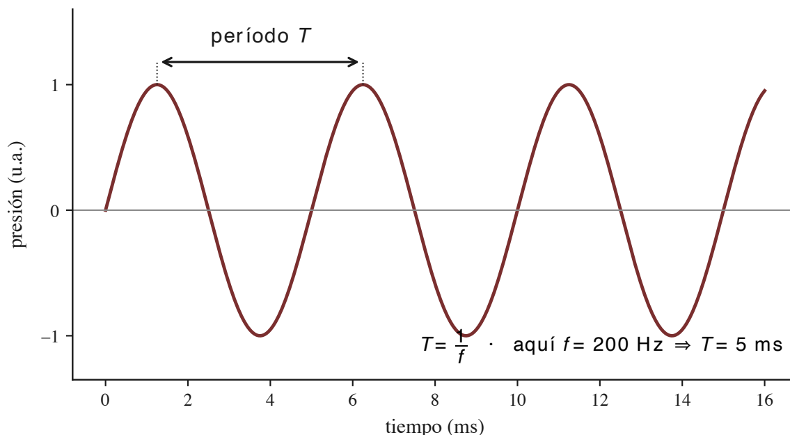
Figura 2: Figura 2. Frecuencia y período, el mismo dato de dos maneras: sobre una oscilación que se repite, T mide cuánto dura un ciclo y f = 1/T cuántos ciclos ocurren por segundo. En el ejemplo, f = 200 \text{ Hz} equivale a T = 5 \text{ ms} .
