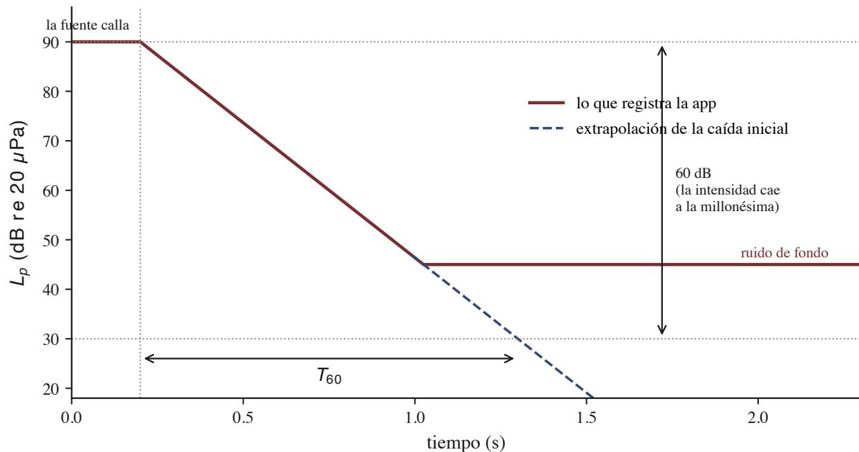
Figura 14: Figura 1. El T_{60} en una gráfica (esquemática): cuando la fuente calla, el nivel cae en línea recta en dB, y el T_{60} es el tiempo en bajar 60 dB — seis pisos de \times 10 . En una medición real la cola se funde con el ruido de fondo antes de completar la caída: se lee la pendiente inicial y se extrapola. Exactamente lo que haremos en la salida.
