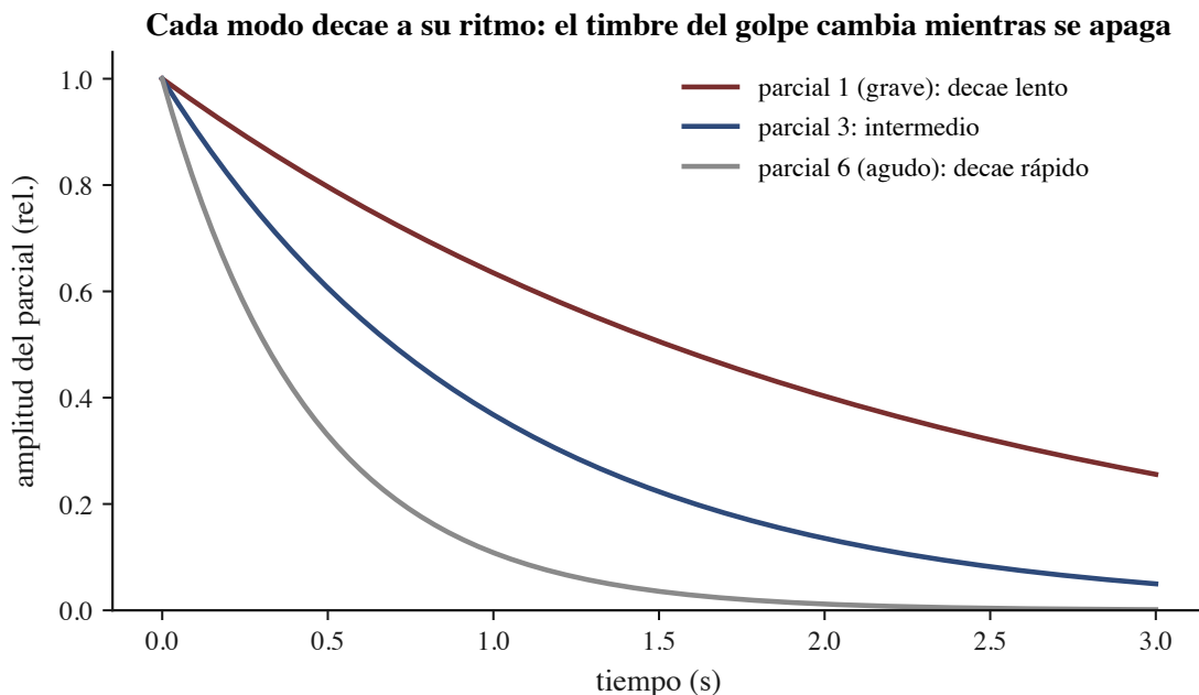
Figura 3: Figura 2. Los modos de un objeto golpeado no mueren juntos: en general los agudos se apagan antes que los graves. Como la mezcla de parciales cambia con el tiempo, el timbre de un golpe es una película —brillante al principio, más simple hacia la cola—, no una foto. Curvas esquemáticas.
