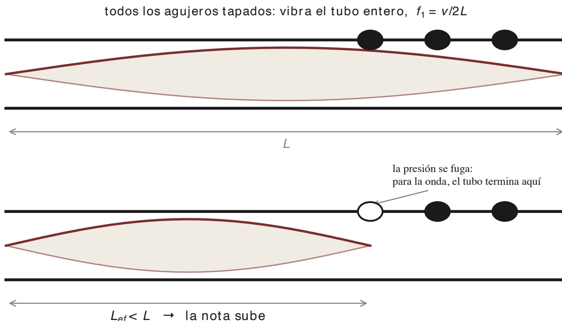
Figura 12: Figura 2. Un agujero abierto es una fuga de presión: para la onda, el tubo termina aproximadamente donde está el primer agujero destapado (esquemático). El largo efectivo L_{ef} es menor que L y la nota sube.
