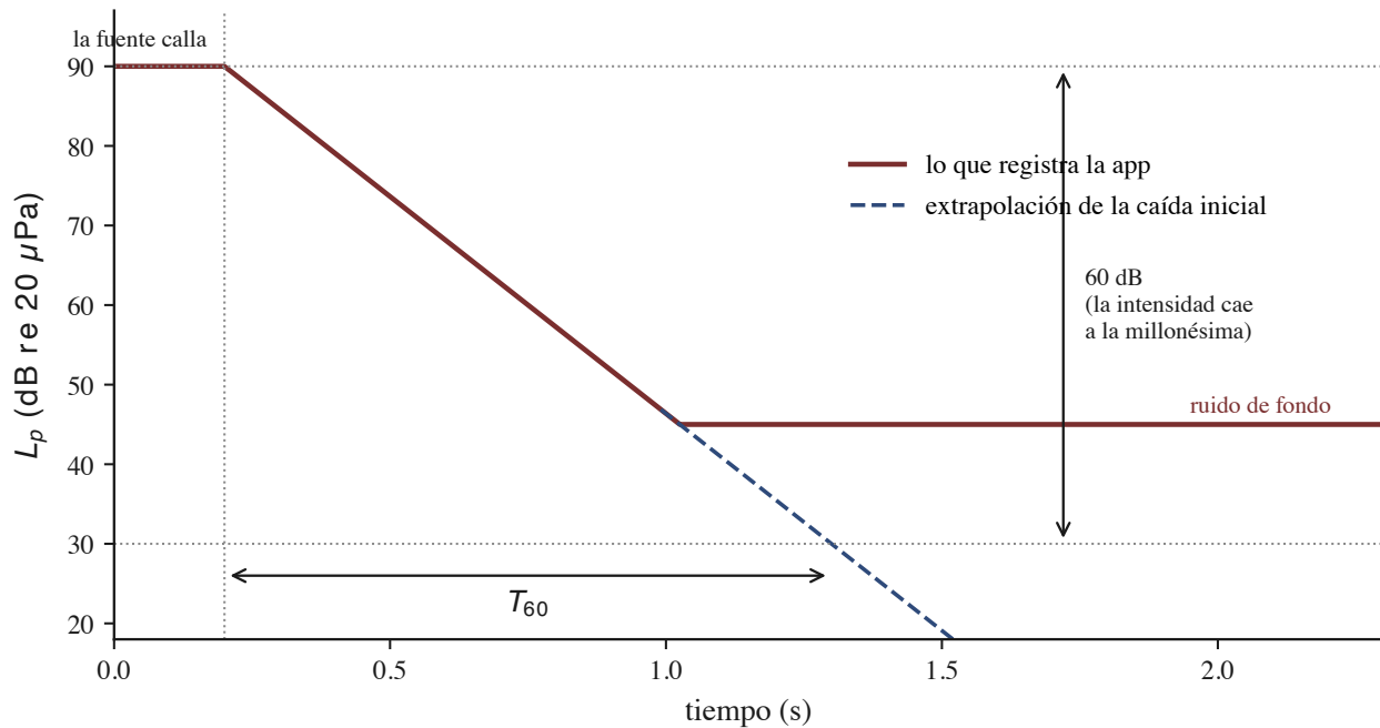
Figura 1. El T_{60} en una gráfica (esquemática): cuando la fuente calla, el nivel cae en línea recta en dB, y el T_{60} es el tiempo en bajar 60 dB — seis pisos de \times 10 . En una medición real la cola se funde con el ruido de fondo antes de completar la caída: se lee la pendiente inicial y se extrapola. Exactamente lo que haremos en la salida.
