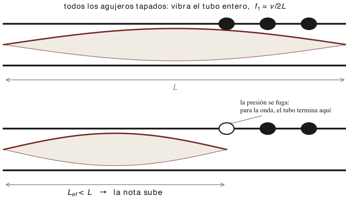
Figura 2. Un agujero abierto es una fuga de presión: para la onda, el tubo termina aproximadamente donde está el primer agujero destapado (esquemático). El largo efectivo L_{ef} es menor que L y la nota sube.
