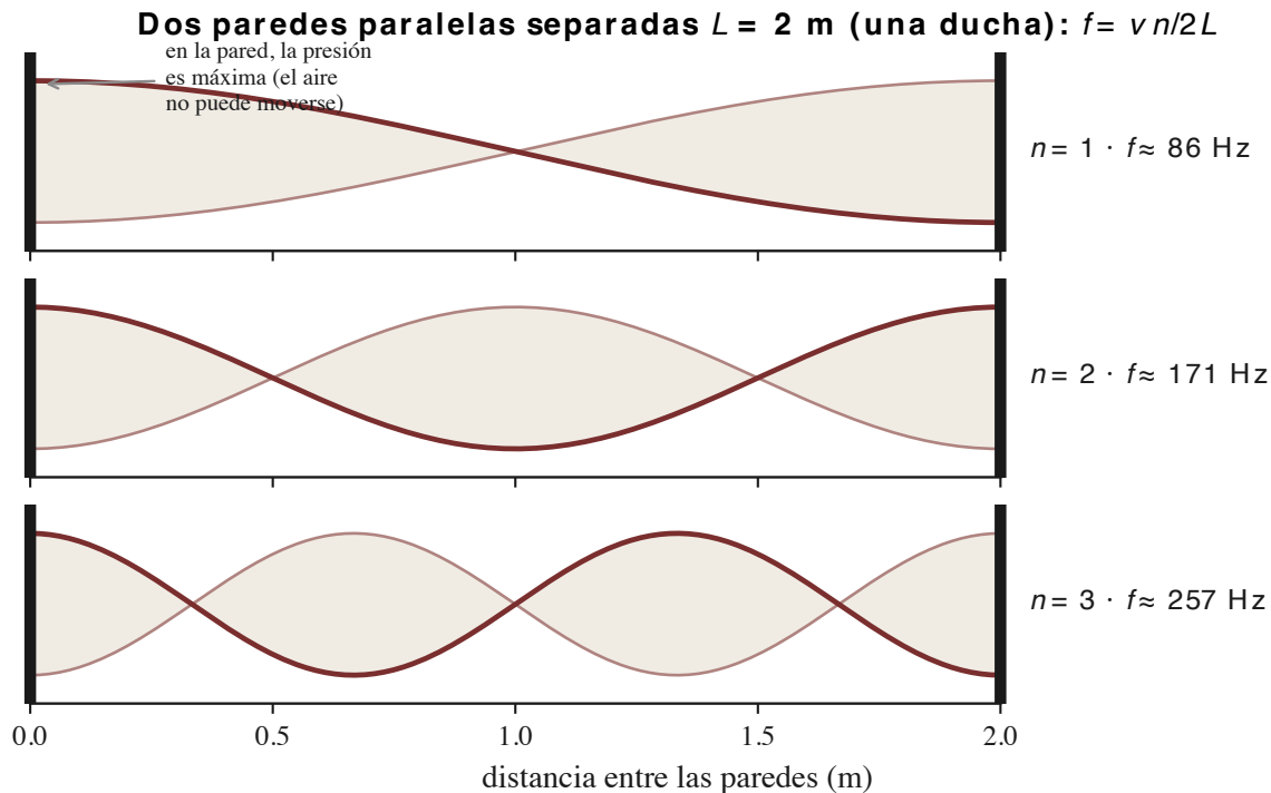
Figura 2. Los tres primeros modos axiales entre dos paredes separadas L = 2 m: f = v n / 2L \approx 86 , 171 y 257 Hz. En la pared rígida el aire no puede moverse y la presión es máxima — al revés que en el extremo abierto de los tubos de s12. Pocos modos, bien separados, en plena zona de la voz: por eso la ducha tiene favoritas.
