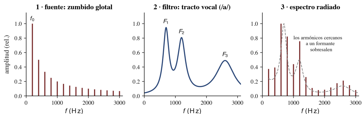
Figura 1. El modelo fuente-filtro en tres pasos (esquemático; una /a/ con f_0 = 200 Hz): el zumbido glotal pone el peine de armónicos, el tracto pone la envolvente de formantes, y lo radiado es el producto de ambos. La sesión hará este experimento en vivo, con su voz y el espectrograma proyectado.
