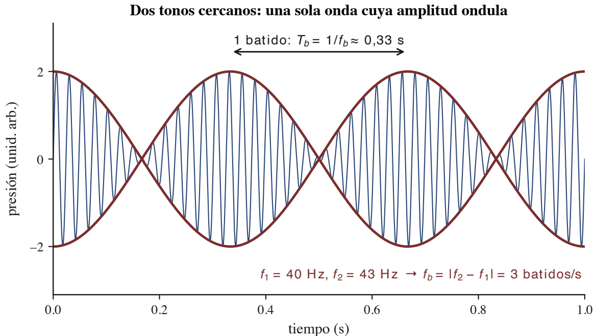
Figura 1. Suma de dos tonos cercanos: una onda rápida (a la frecuencia promedio) encerrada por una envolvente lenta (rojo) que sube y baja f_b = |f_2 - f_1| veces por segundo — refuerzo, silencio, refuerzo. Se dibuja con f_1 = 40 \text{ Hz} y f_2 = 43 \text{ Hz} para que el ciclo sea visible.
