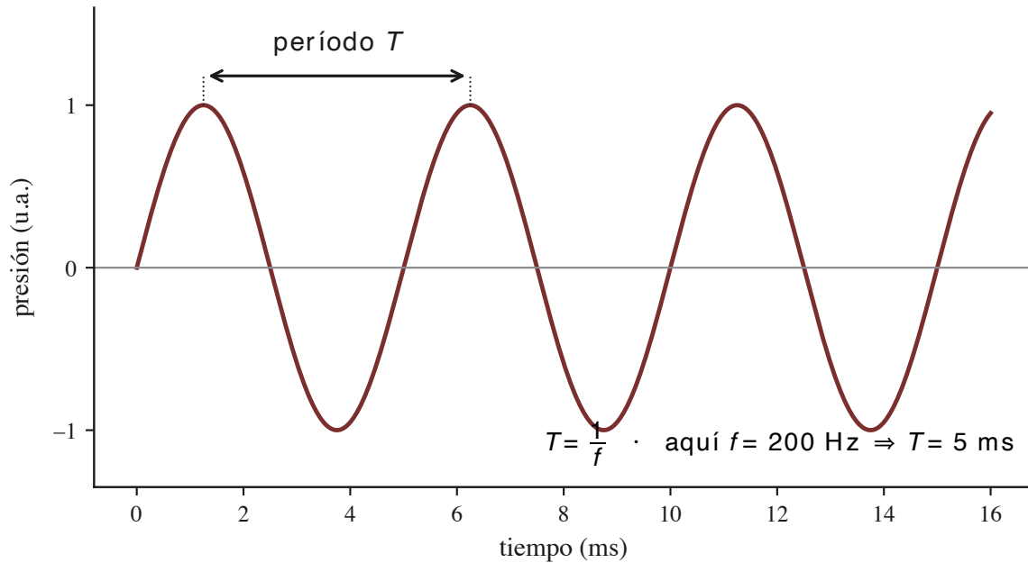
Figura 2. Frecuencia y período, el mismo dato de dos maneras: sobre una oscilación que se repite, T mide cuánto dura un ciclo y f = 1/T cuántos ciclos ocurren por segundo. En el ejemplo, f = 200 \text{ Hz} equivale a T = 5 \text{ ms} .
