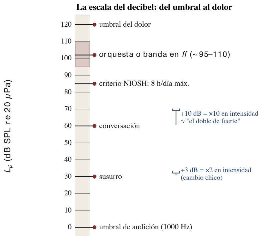
Figura 1. La escala de niveles de presión sonora con hitos musicales, del umbral de audición al umbral del dolor. Los valores son típicos y redondeados. A la derecha, la gramática del decibel: +10 dB multiplican por diez la intensidad (y suenan como el doble), +3 dB la duplican (cambio chico).
