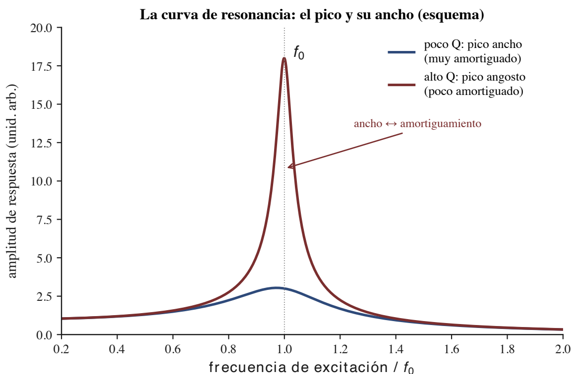
Figura 1. La curva de respuesta de un resonador (esquema): cuánto responde frente a la frecuencia con que se lo fuerza, con un pico en su frecuencia propia f_0 . Poco amortiguamiento da un pico alto y angosto (la copa de cristal, que exige su nota exacta); mucho amortiguamiento da un pico bajo y ancho (responde algo a muchas frecuencias vecinas).
