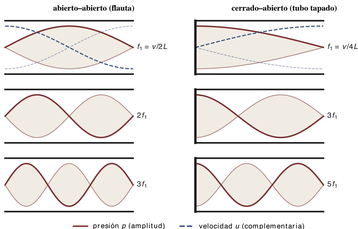
Figura 1. Amplitud de la onda estacionaria de presión de los tres primeros modos de un tubo abierto–abierto y de uno cerrado–abierto. La “puerta” (extremo abierto) impone un nodo de presión; la “pared” (tapa), un máximo. La velocidad del aire (punteada, primera fila) es complementaria: máxima donde la presión tiene nodo. Entre puerta y pared cabe solo un cuarto de onda: de ahí el 4L y la serie impar.
