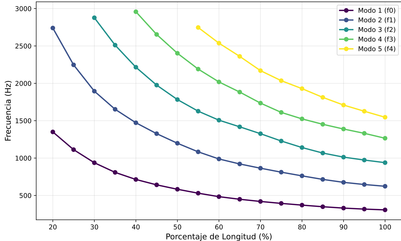
Frecuencias de Resonancia vs. Longitud Truncada Deppe
