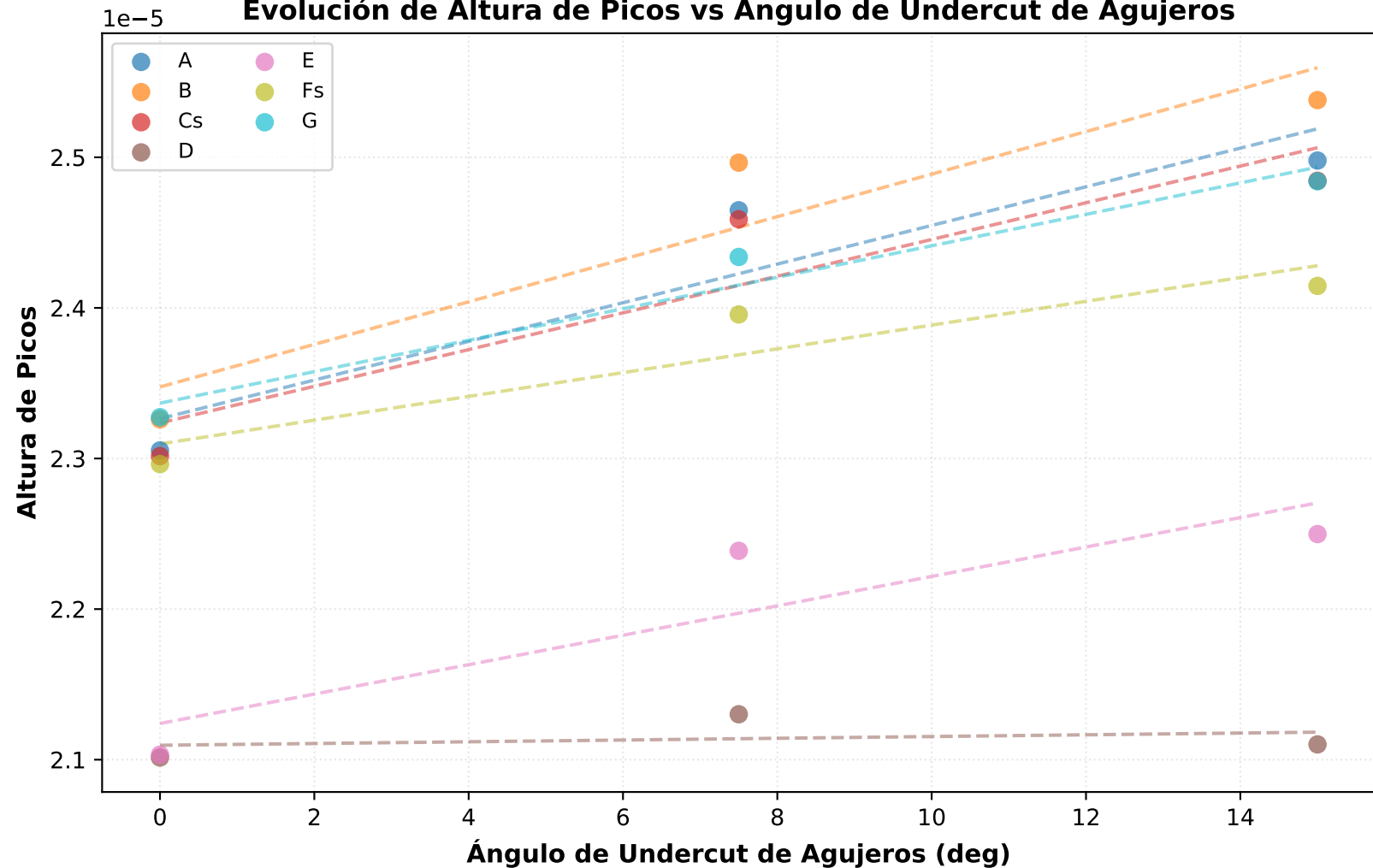
Evolución de Altura de Picos vs Ángulo de Undercut de Agujeros
