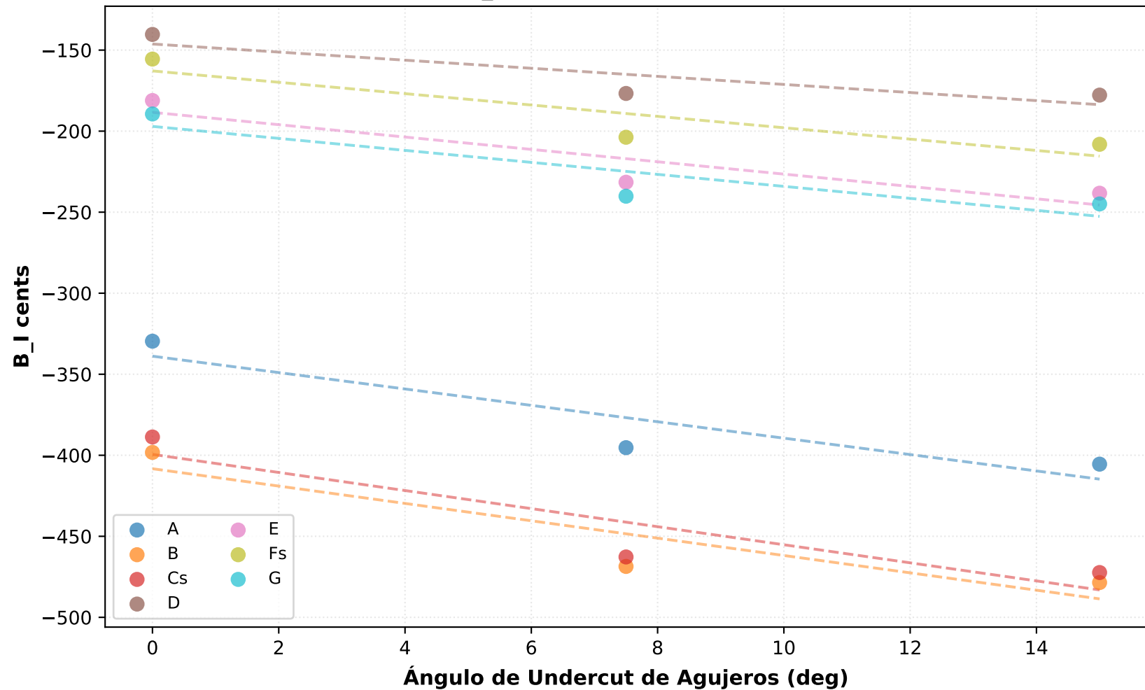
Evolución de B_I vs Ángulo de Undercut de Agujeros
