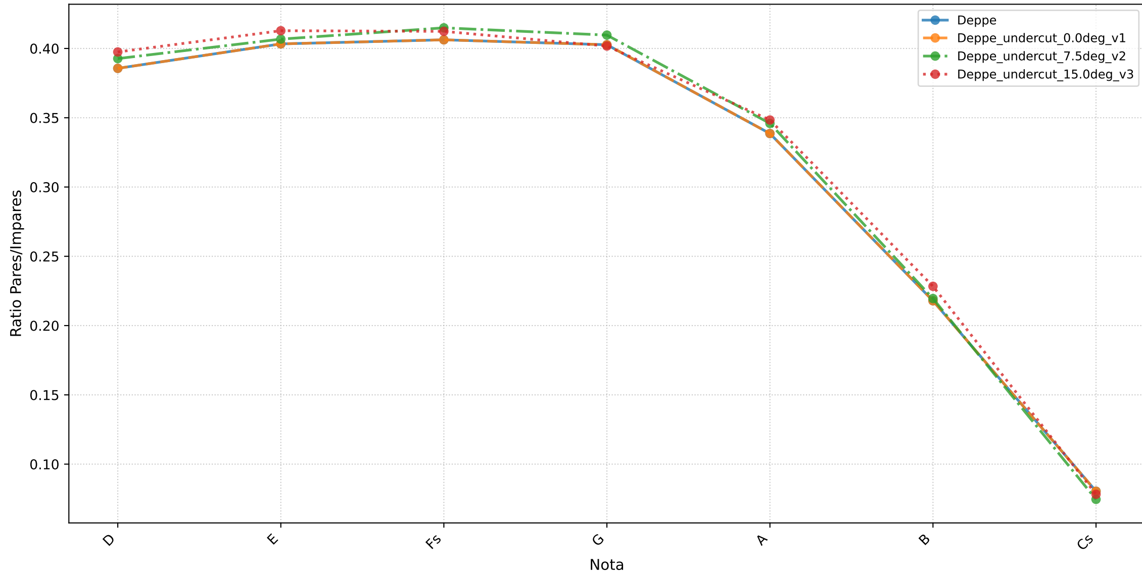
Ratio de Armónicos Pares/Impares (Carácter Tonal)
