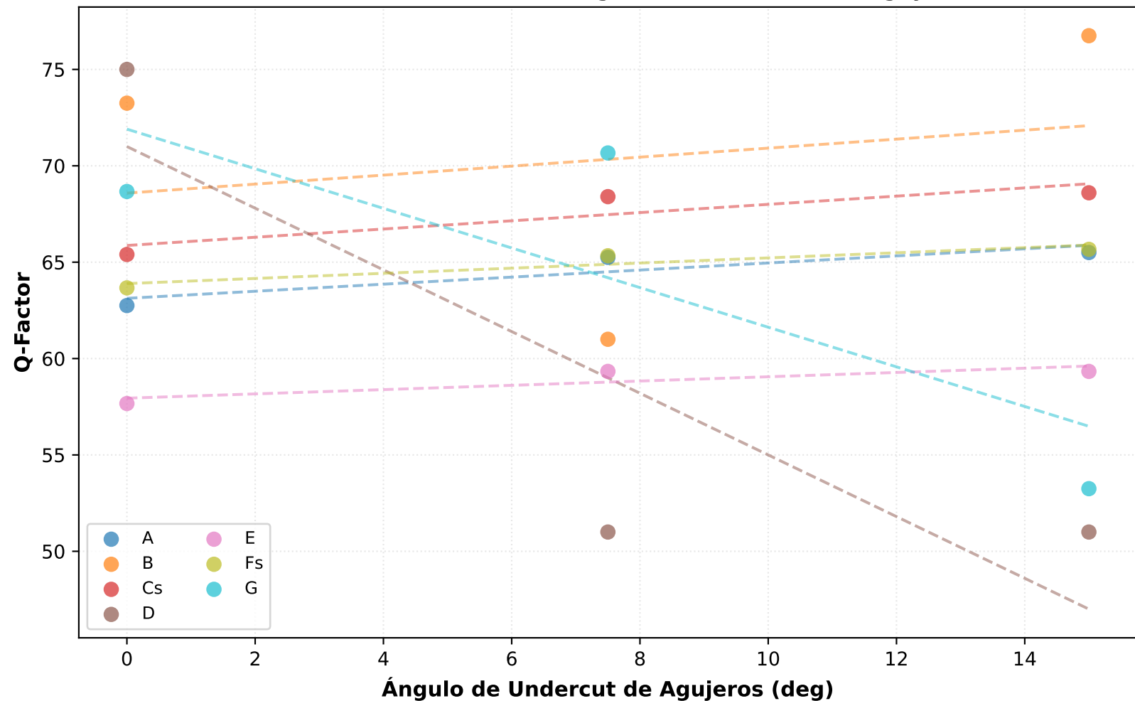
Evolución de Q-Factor vs Ángulo de Undercut de Agujeros
