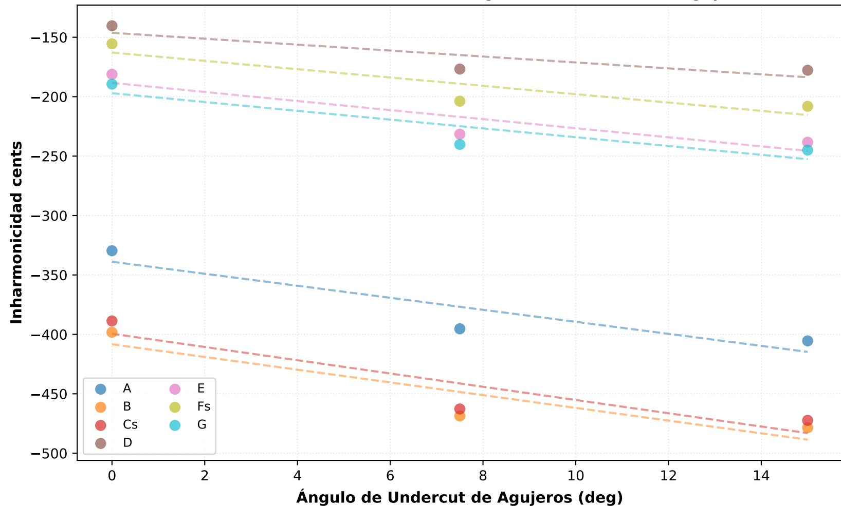
Evolución de Inharmonicidad vs Ángulo de Undercut de Agujeros
