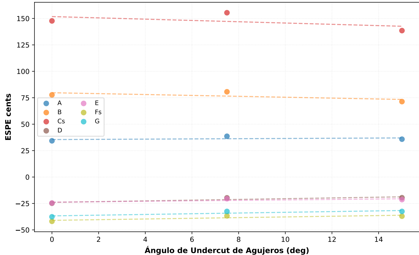
Evolución de ESPE vs Ángulo de Undercut de Agujeros
