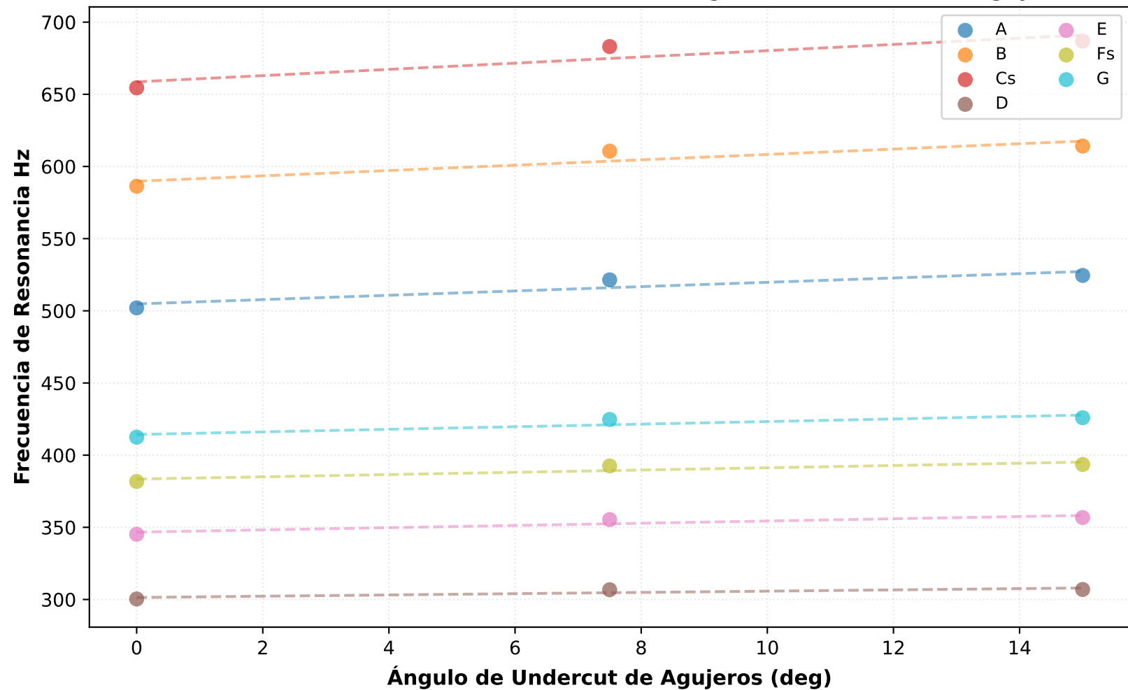
Evolución de Frecuencia de Resonancia vs Ángulo de Undercut de Agujeros
