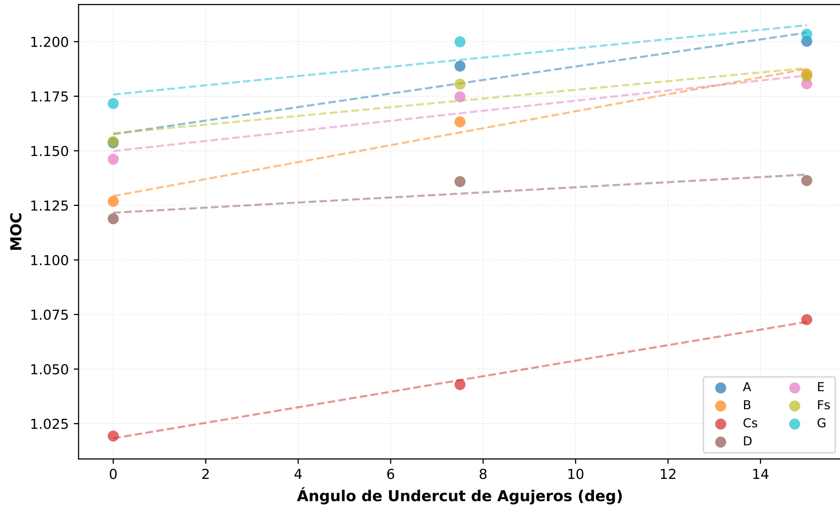
Evolución de MOC vs Ángulo de Undercut de Agujeros
