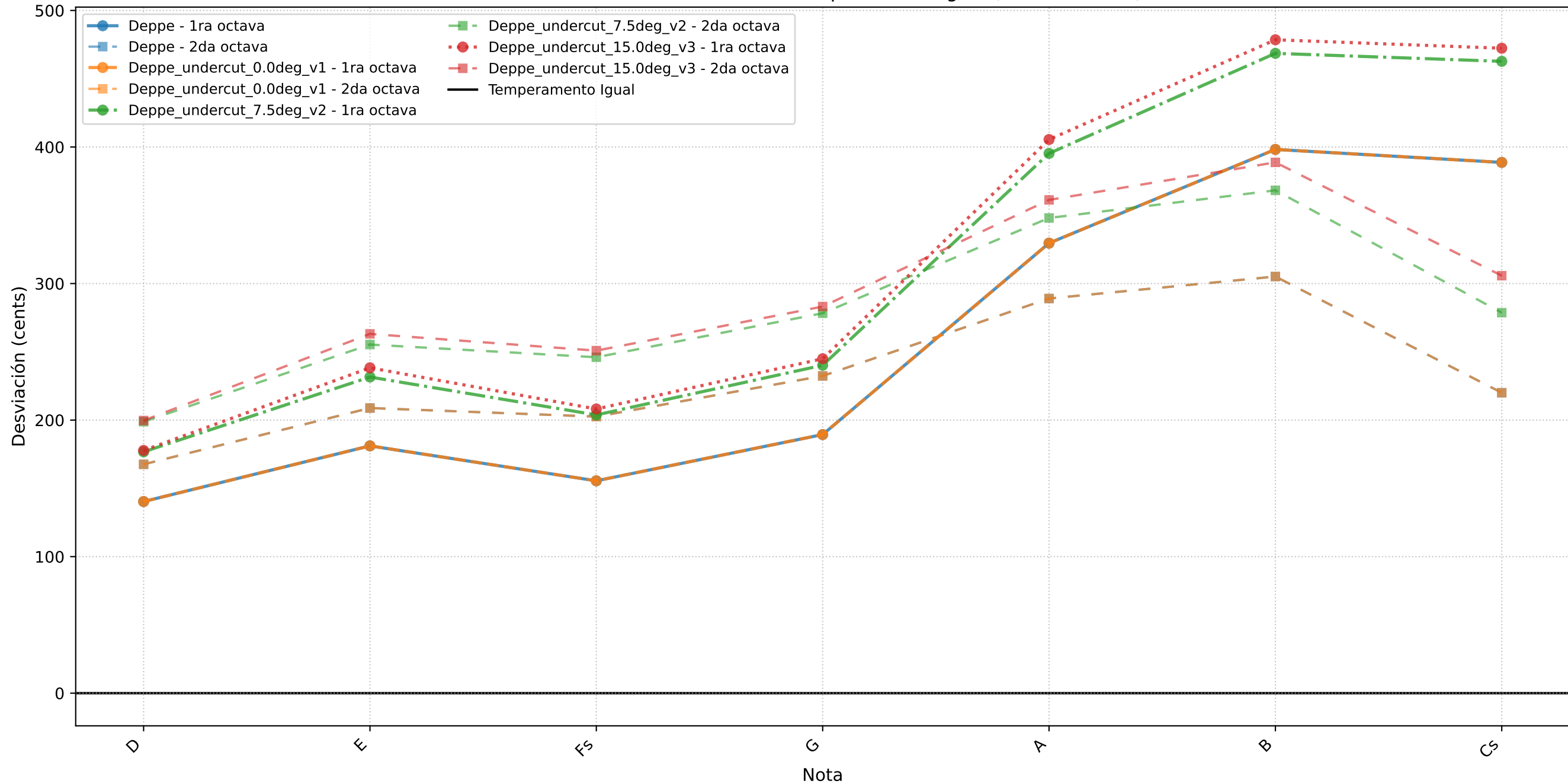
Frecuencias de Resonancia vs Temperamento Igual (La = 415.0 Hz)
