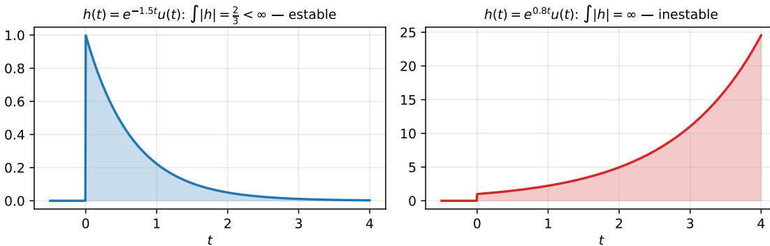
Figura 2.6: La estabilidad se ve en el área bajo |h| : si es finita (izquierda), ninguna entrada acotada puede hacer explotar la salida; si diverge (derecha), el sistema explota incluso solo.
