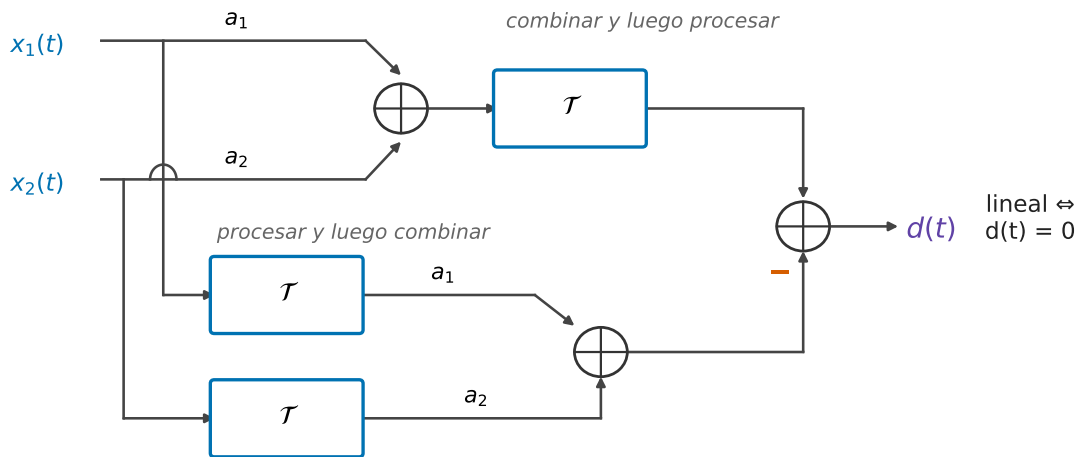
Figura 2.1: El test de linealidad como diagrama de bloques. Camino de arriba: las entradas se combinan primero (con pesos a_1 y a_2 ) y la mezcla entra al sistema. Camino de abajo: cada entrada pasa por su propia copia del sistema y recién después se combinan, con los mismos pesos. El nodo final resta ambos resultados. El sistema es lineal si y solo si d(t) = 0 para toda entrada y todo par de pesos. Nota: el arco sobre la línea de x_2 indica que ese cable cruza sin conectarse.
