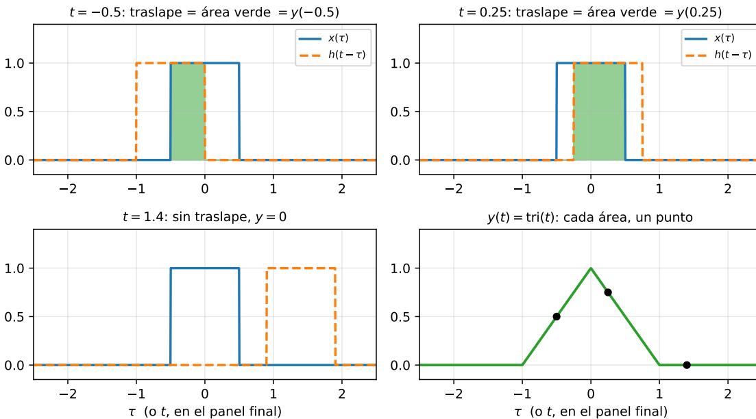
Figura 2.4: El método gráfico en acción para \text{rect} * \text{rect} . En cada instante t , la ventana invertida h(t-\tau) se desplaza sobre x(\tau) ; el área del producto (verde) es un único número, y(t) . El panel final reúne todos esos números: el triángulo.
