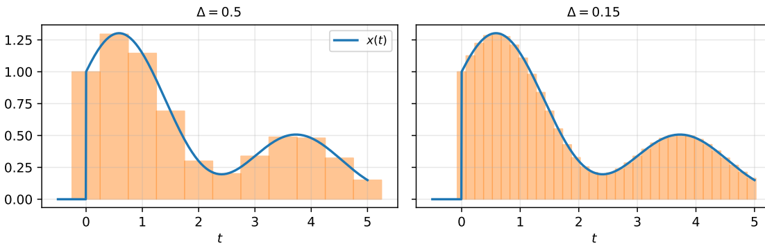
Figura 2.3: La escalera de pulsos que aproxima a x(t) . Al afinar \Delta , los pulsos se vuelven impulsos, la suma se vuelve integral, y la aproximación se vuelve identidad: toda señal es una suma continua de impulsos pesados.
