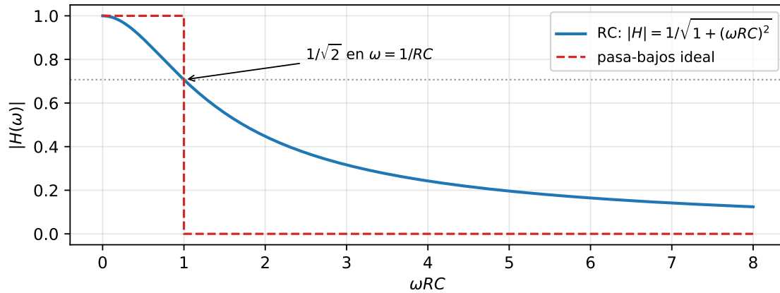
Figura 3.5: Respuesta en frecuencia del filtro RC (pasa-bajos real) y del pasa-bajos ideal con el mismo corte. El ideal corta en seco; el RC negocia una transición gradual — y a cambio existe.
