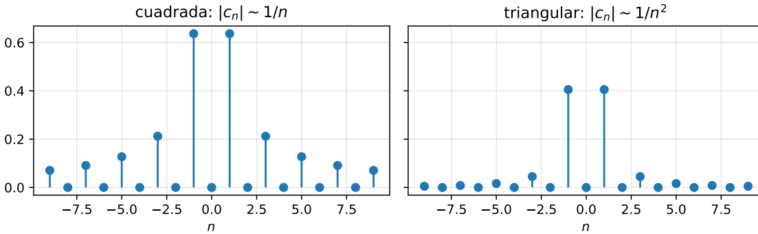
Figura 3.2: Espectros de línea: |c_n| de la onda cuadrada (decae como 1/n : tiene saltos) y de la triangular (decae como 1/n^2 : continua, con puntas). Mirar cómo decae el espectro es mirar cuán suave es la señal.
