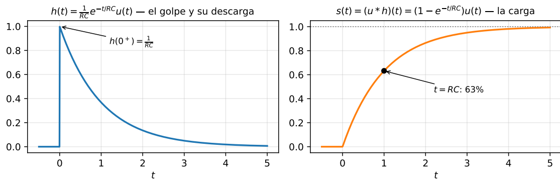
Figura 2.5: El sistema RC visto desde sus dos respuestas: al impulso (izquierda, salta a 1/RC y se descarga) y al escalón (derecha, la curva de carga del condensador). Están conectadas: s' = h .
