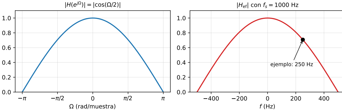
Figura 5.6: El mismo filtro, dos rectas de medir. Izquierda: |H(e^{j\Omega})| del promedio móvil en el eje discreto (periódica en 2\pi , cero en \Omega = \pi ). Derecha: la respuesta efectiva de la cadena con f_s = 1000 Hz — la misma curva con el eje reescalado a Hz; el cero cae en f_s/2 = 500 Hz. El punto marca el ejemplo resuelto (250 Hz).
