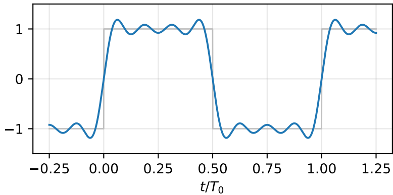
N = 7 armónicos
