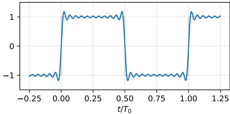
N = 21 armónicos
