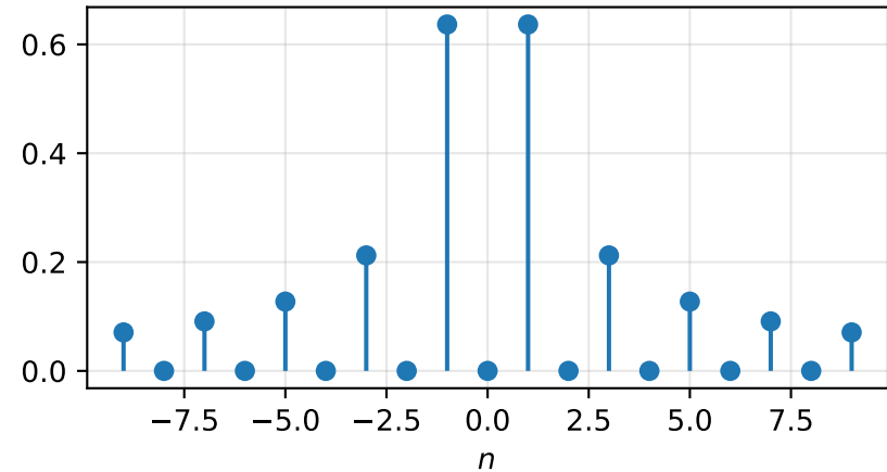
cuadrada: |c_n| \sim 1/n
