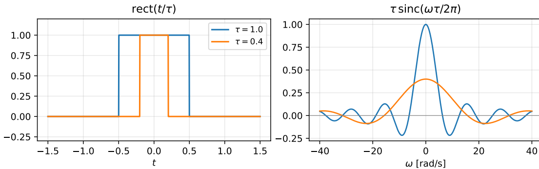
Figura 3.4: El par rect \leftrightarrow sinc para dos anchos de pulso. El pulso angosto (naranja) tiene el primer cero de su espectro más lejos: tiempo corto \leftrightarrow banda ancha.
