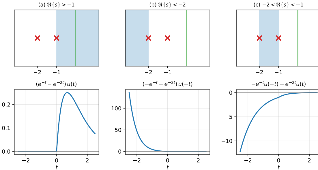
Figura 4.3: Misma fórmula X(s) = 1/((s+1)(s+2)) , tres ROCs, tres señales. Arriba: el plano s con los polos y la ROC de cada caso. Abajo: la señal que corresponde a cada elección.
