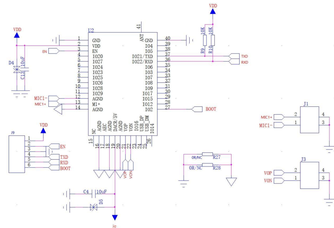
图 11 应用指导电路
