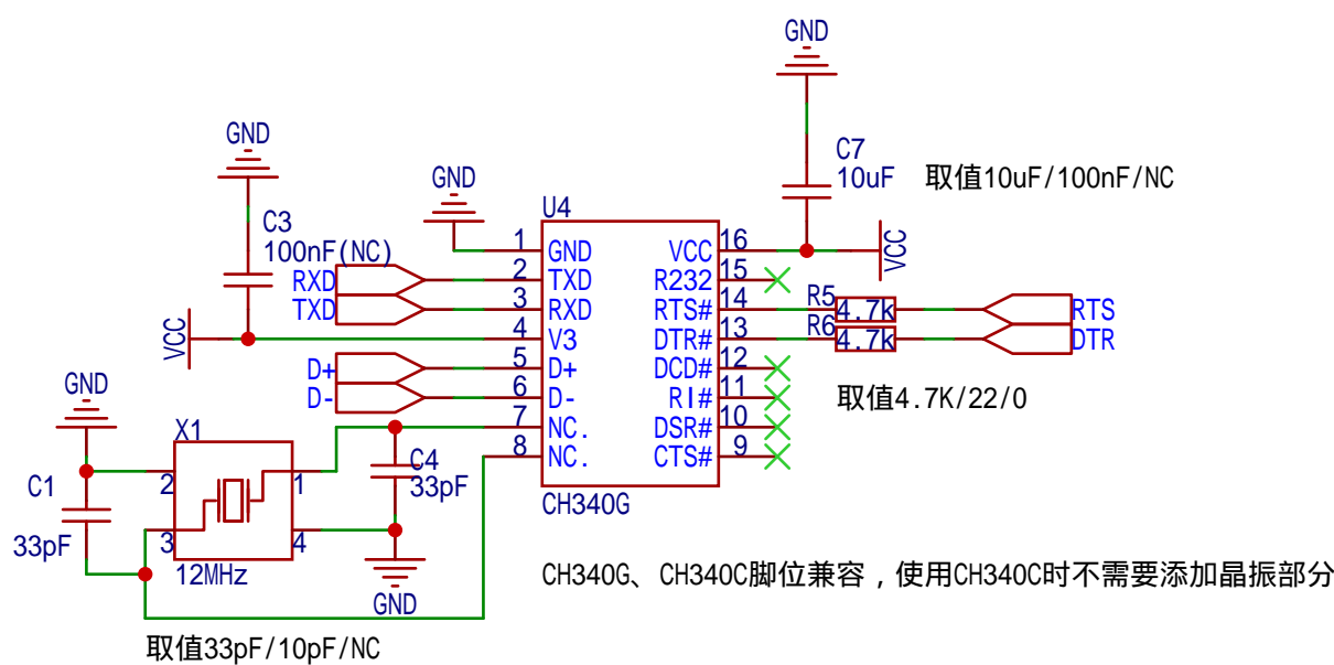
串口电路
