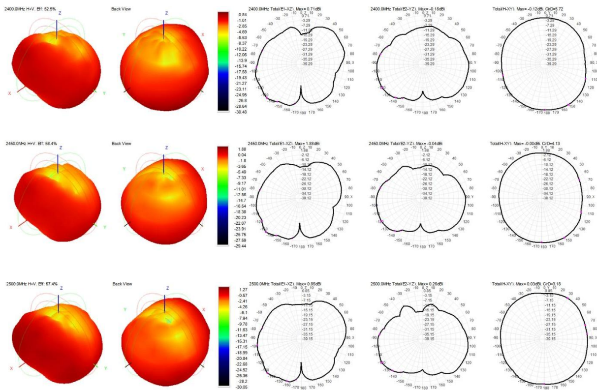
图 10 天线场型图
