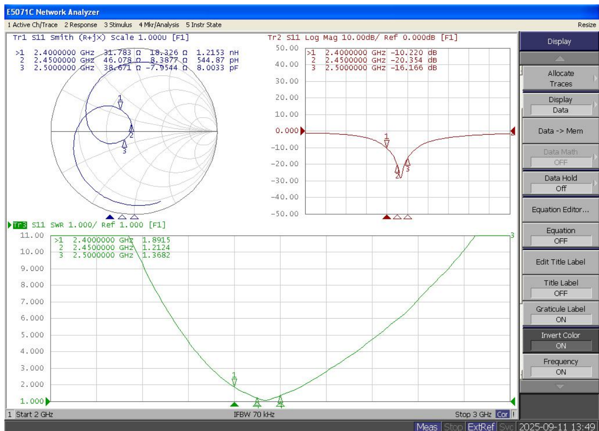
图 9 天线 S 参数
