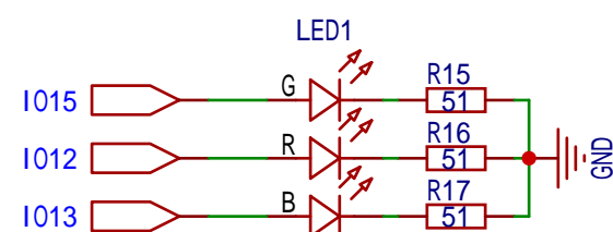
5050 RGB灯
