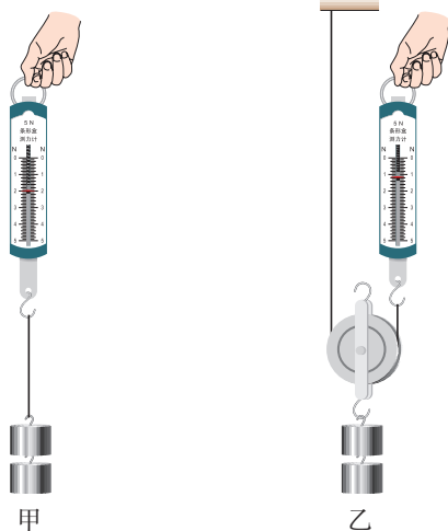
图12.4-1 研究使用动滑轮是否省功
