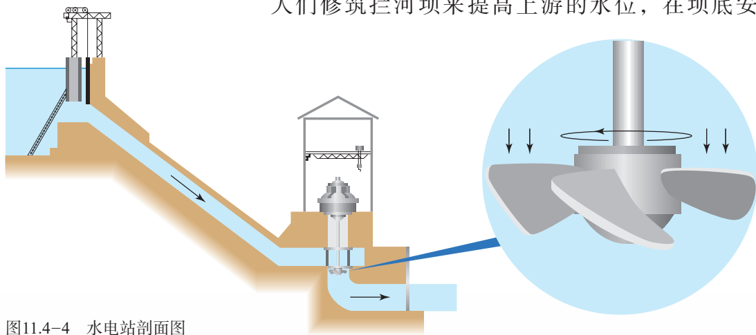
图11.4-4 水电站剖面图
