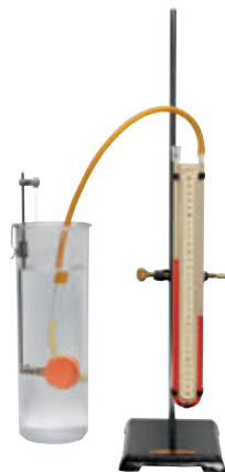
图9.2-2 测量液体压强
