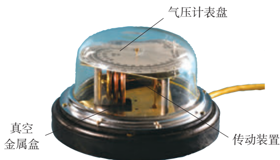
图9.3-4 无液气压计
