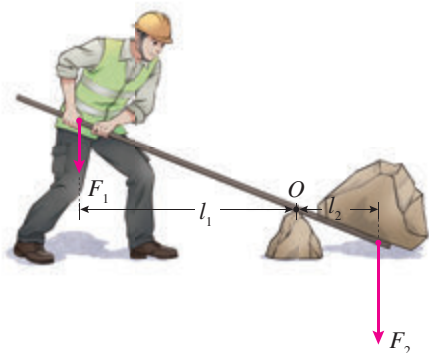
图12.1-2 撬棒
