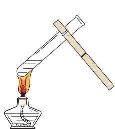
图 1-20 用酒精灯加热 试管中的液体
