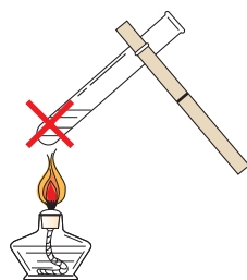
图 1-21 错误的加热操作
