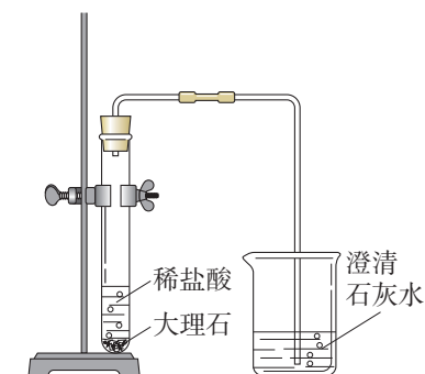
图1-4 大理石与稀盐酸反应
