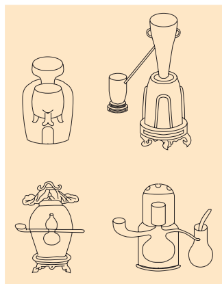
图1-6 中国古代炼丹设备示意图
