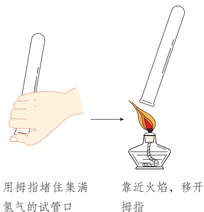
图4-15 检验氢气的纯度
