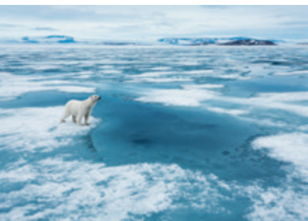
图6-16 全球变暖导致北极熊的栖息地缩小
