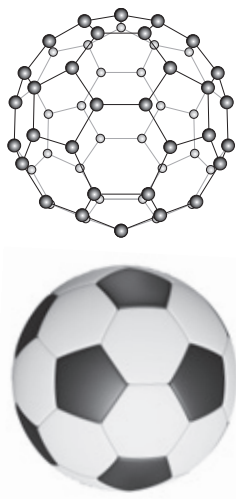
图6-4 C_{60} 的分子结构和足球相似
