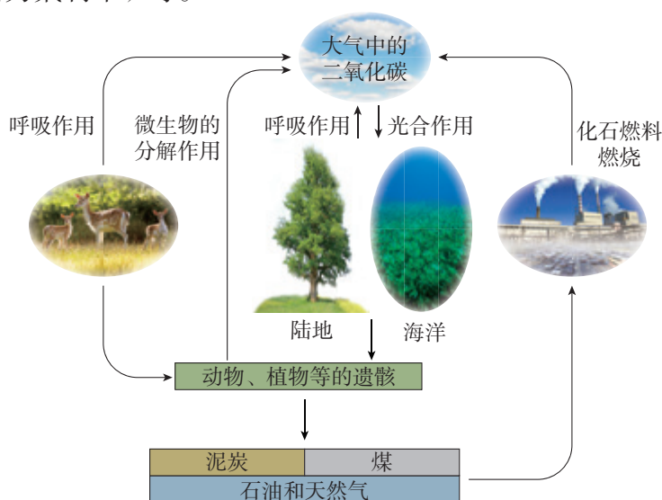
图6-15 自然界中的碳循环示意图（部分）
