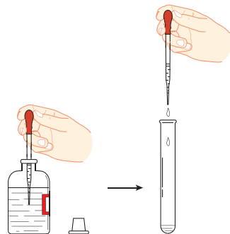
图1-16 用胶头滴管取液体
