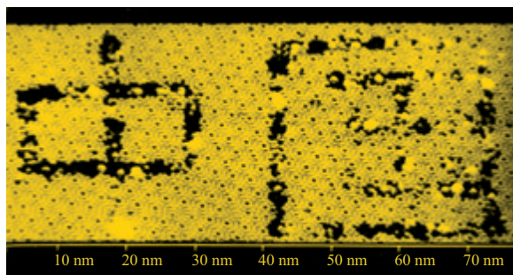
图3-3 通过移走硅原子形成的文字
