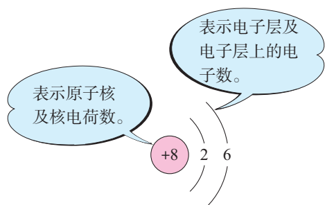
图3-11 氧原子的结构示意图
