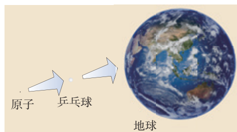
图3-8 原子的体积很小
