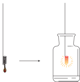
图2-20 铁丝在氧气中燃烧实验示意图
