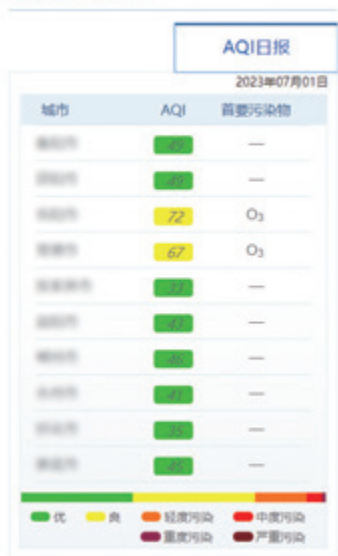
图2-9 空气质量指数日报 （生态环境部发布）
