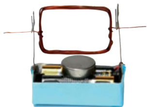
图2 转动的线圈
