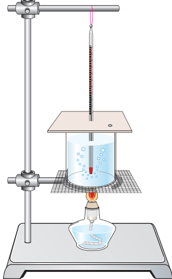
图 3.3-2 观察水沸腾的实验装置
