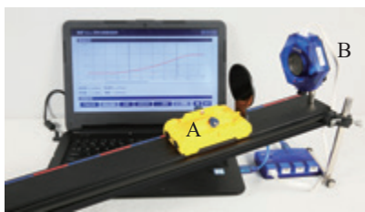
图1.4-3 利用传感器测量物体运动的速度
