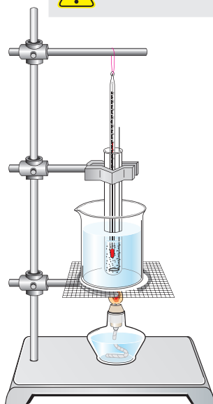
图 3.2-2 观察熔化现象的实验装置
