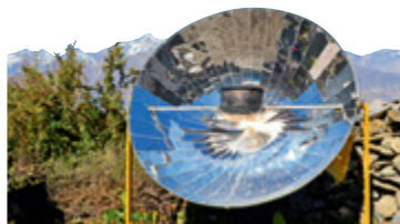
图4.3-8 利用太阳灶煮饭
