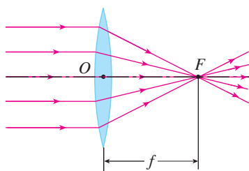
图5.1-7 凸透镜的焦点和焦距
