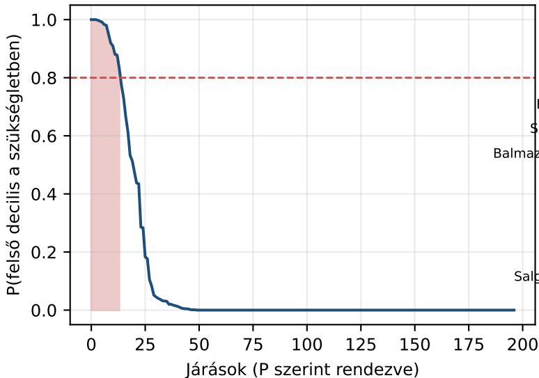
Dirichlet-súlyújramintavétel
