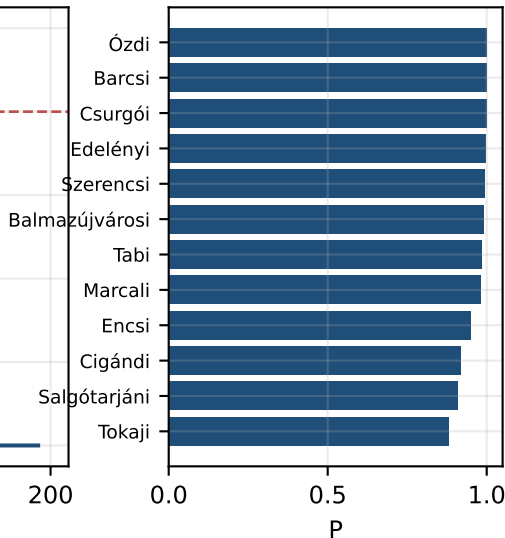
Robusztus prioritás
