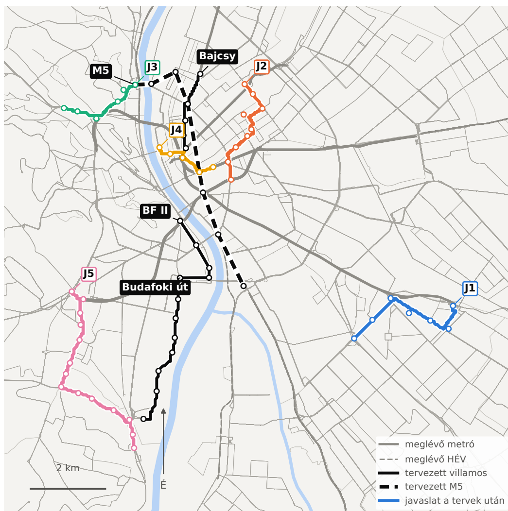
3. ábra. A tervezett fejlesztések (fekete) és a megvalósulásuk utáni legjobb további vonalak (J1–J5, színes) a meglévő kötőtpályás hálózaton.
