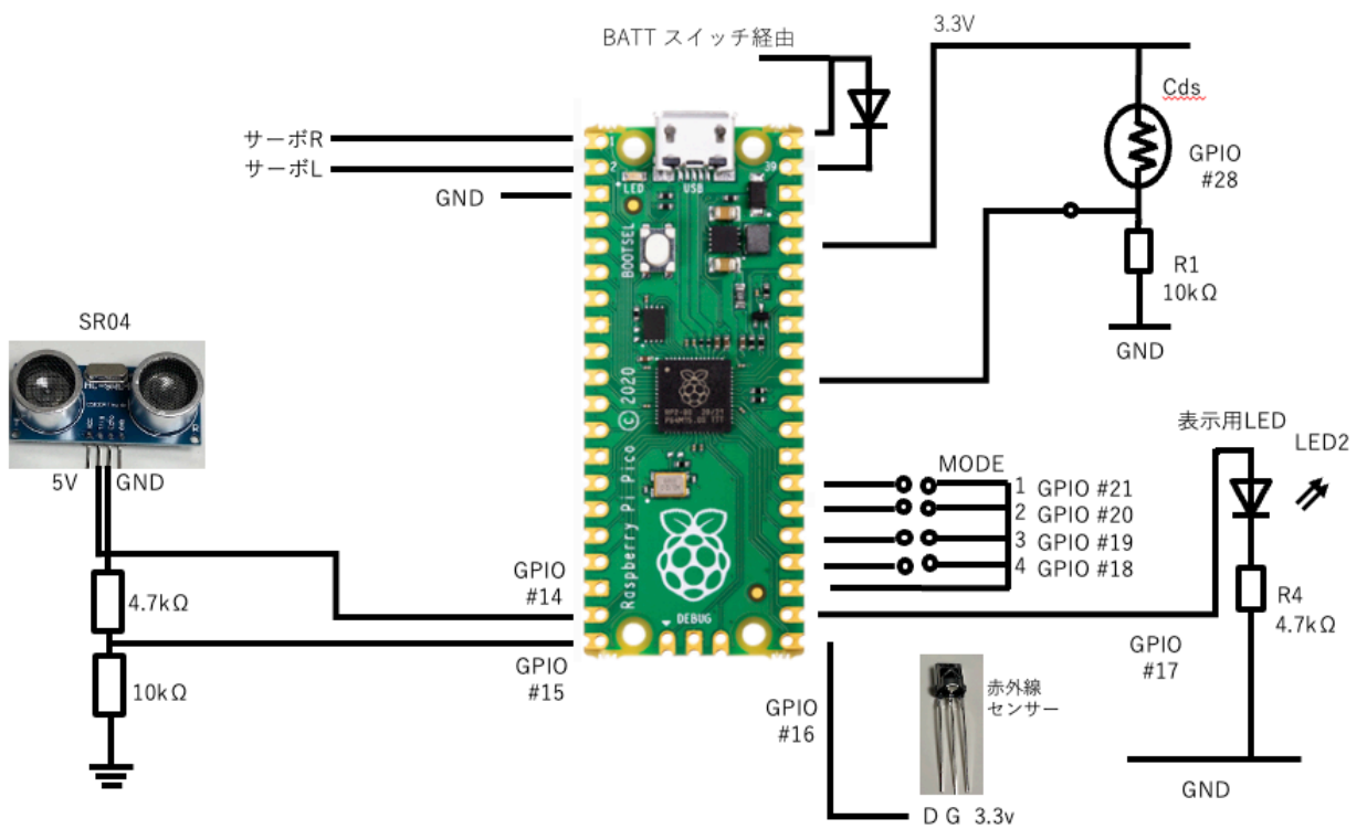
回路図 picoCar v1.0
