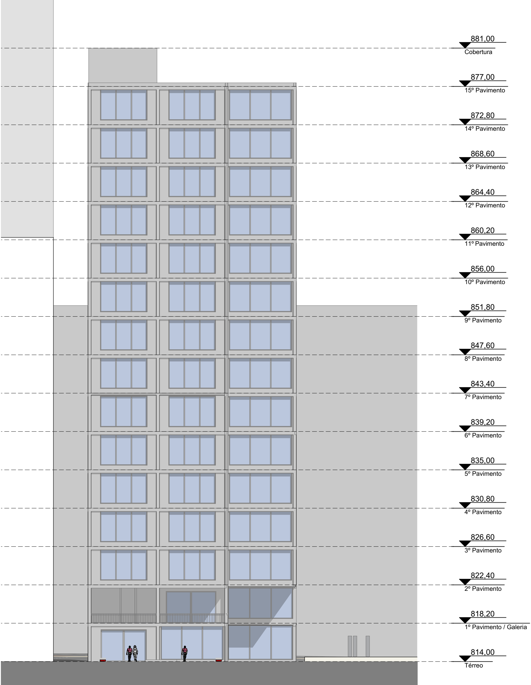
03 POSTERIOR 1:250
