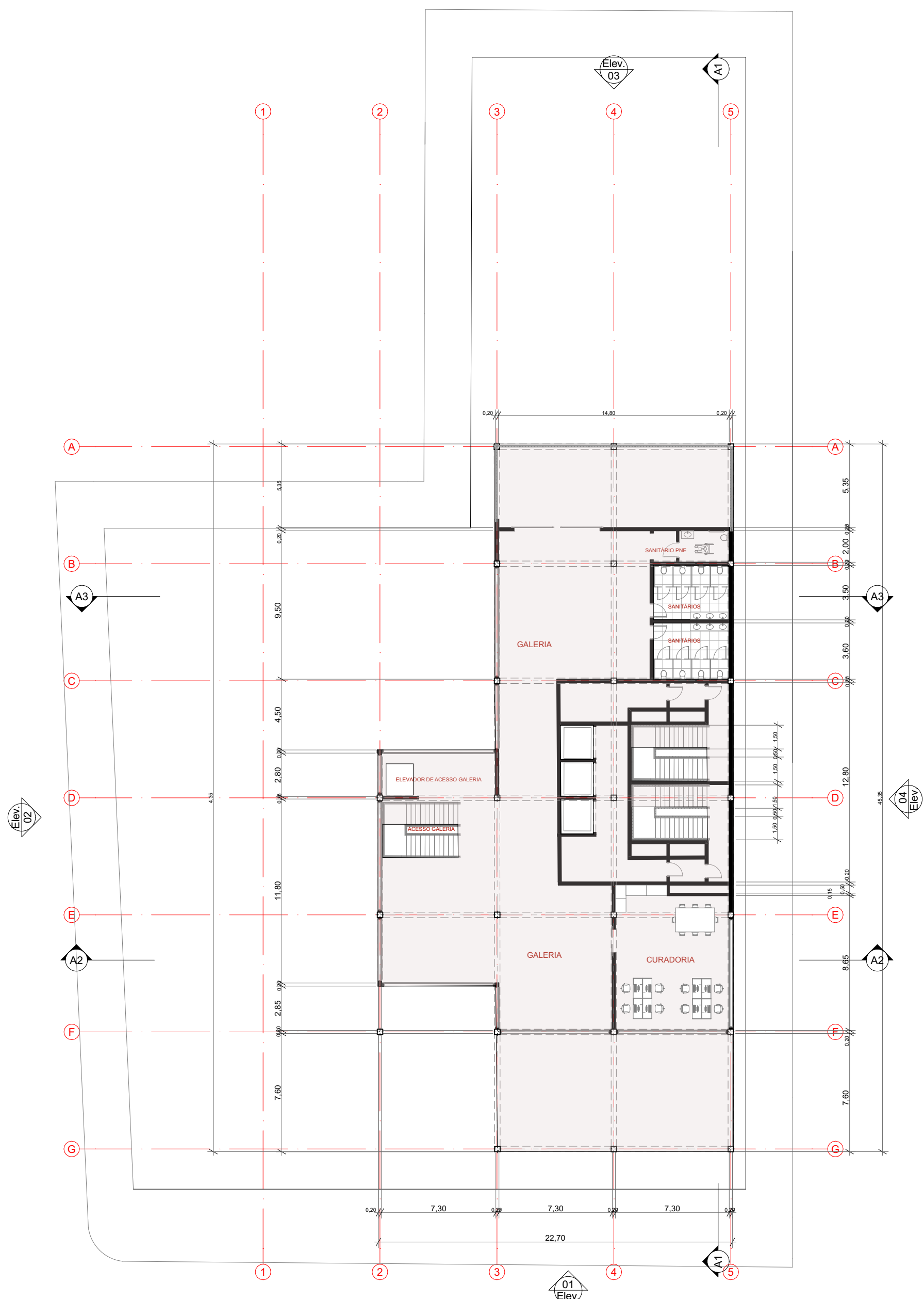
2 PAVIMENTO GALERIA 1:250
