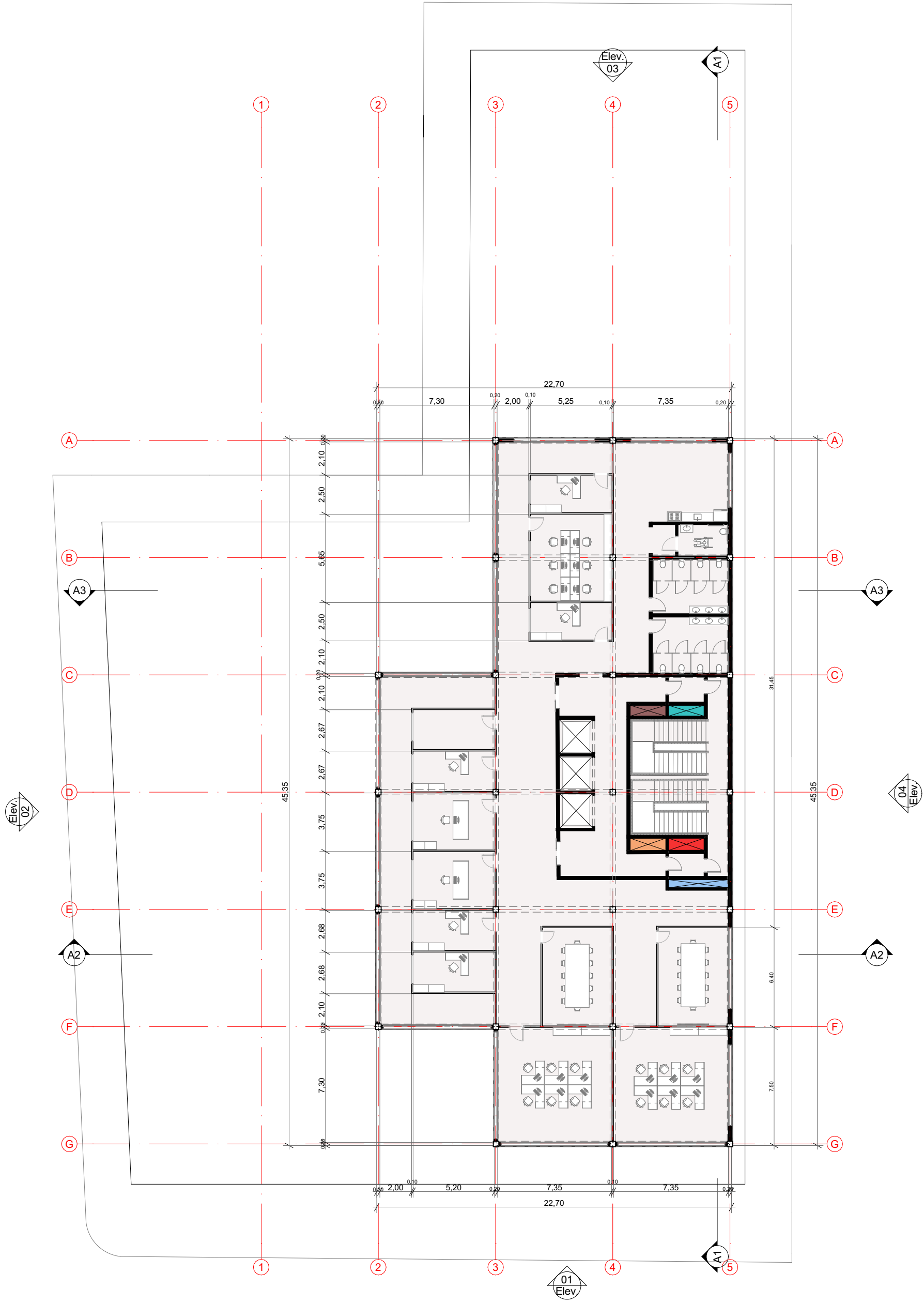
PAVIMENTO TIPO 2 1:250
