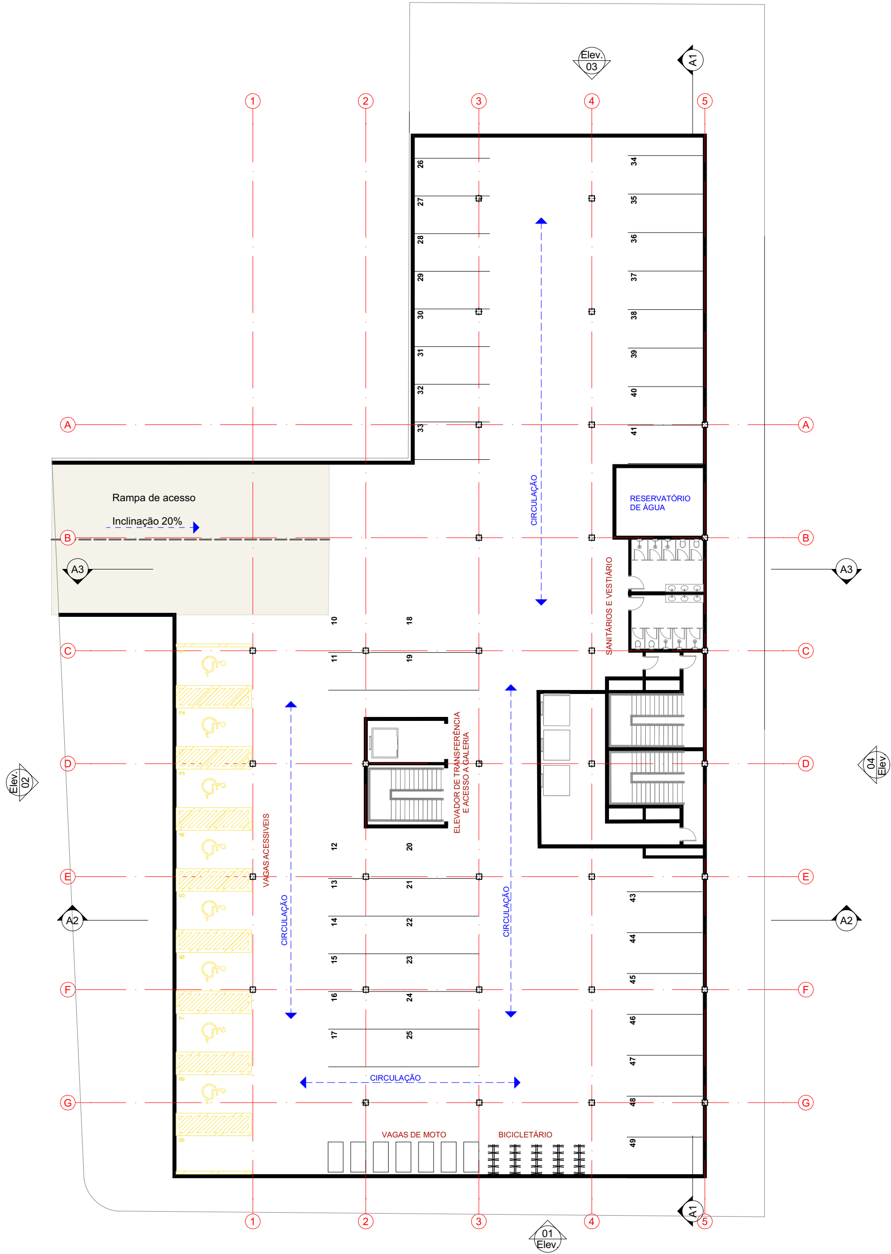
1 PAVIMENTO ESTACIONAMENTO 1:250
