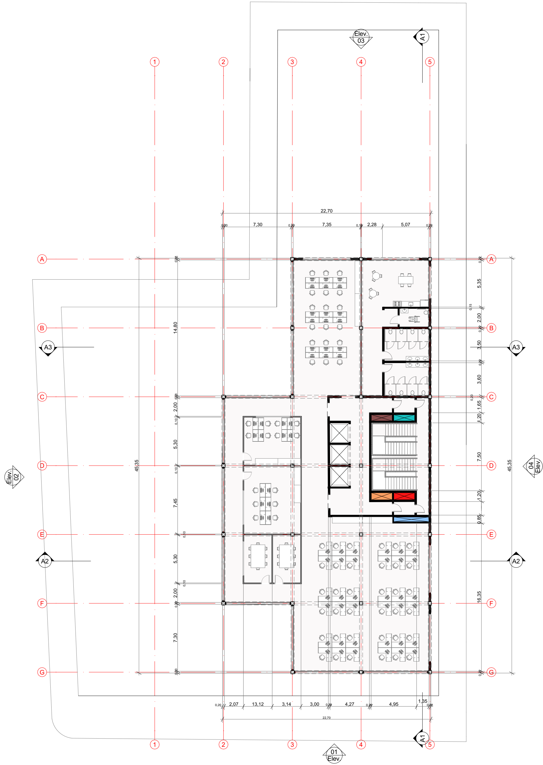
PAVIMENTO TIPO 1 1:250
