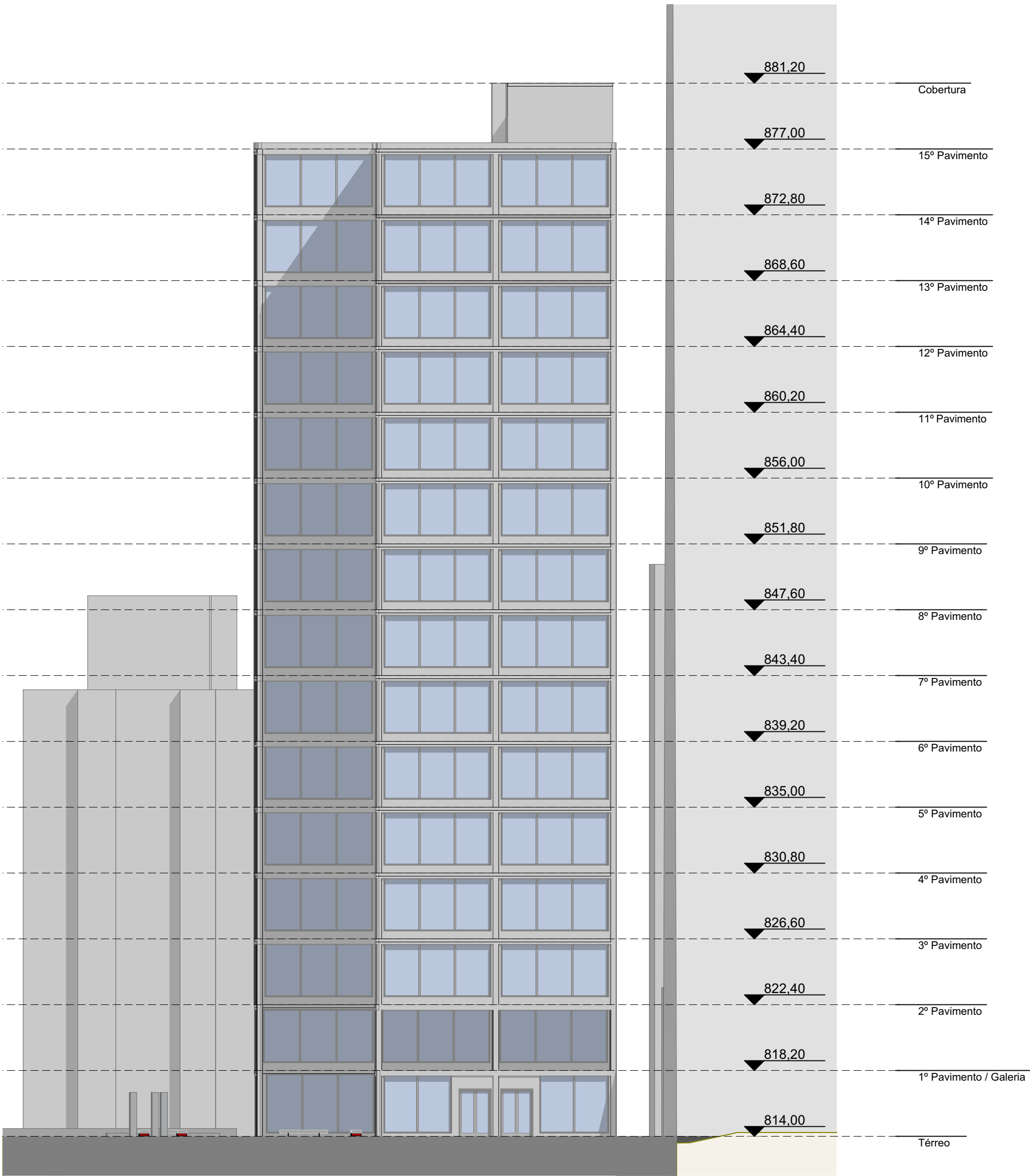
01 ELEVÇÃO FRETE 1:250
