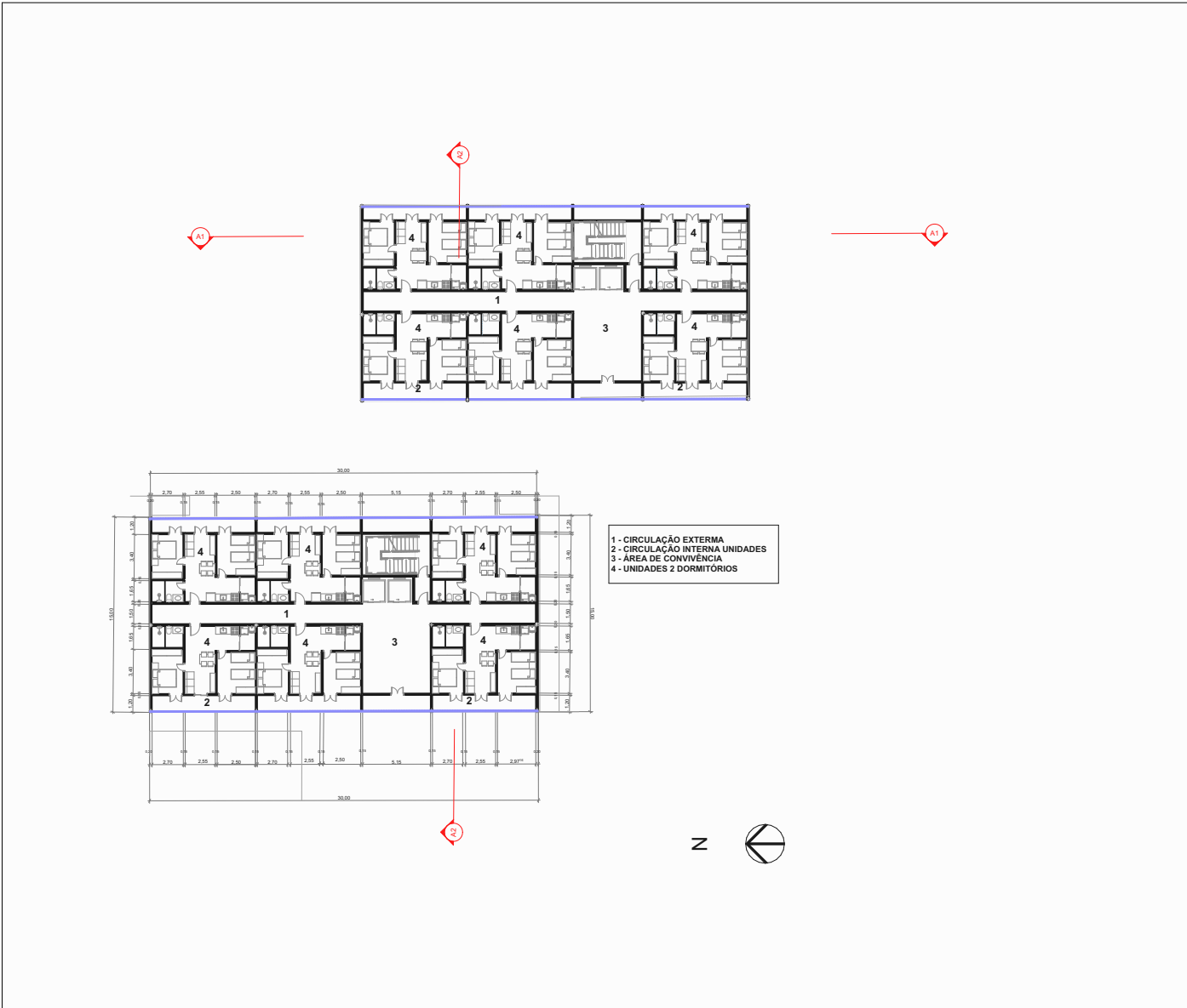
04 PAVIMENTO TIPO 1:500
