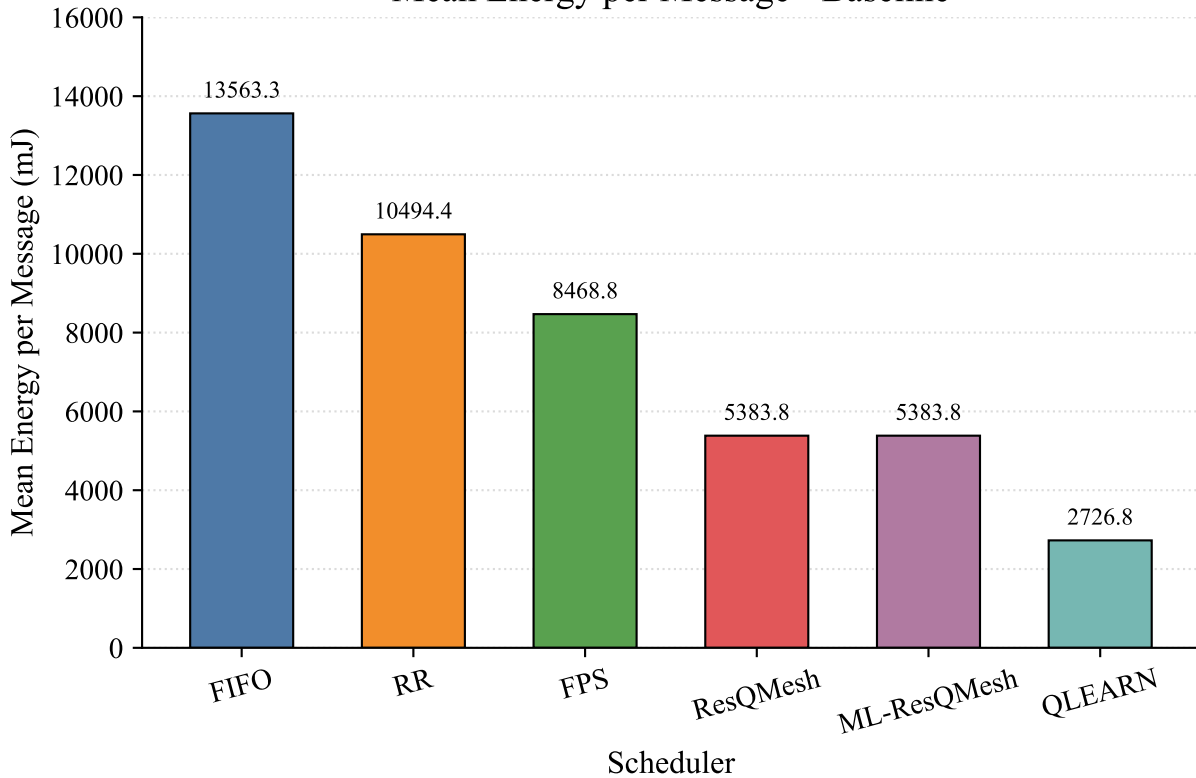
Mean Energy per Message - Baseline
