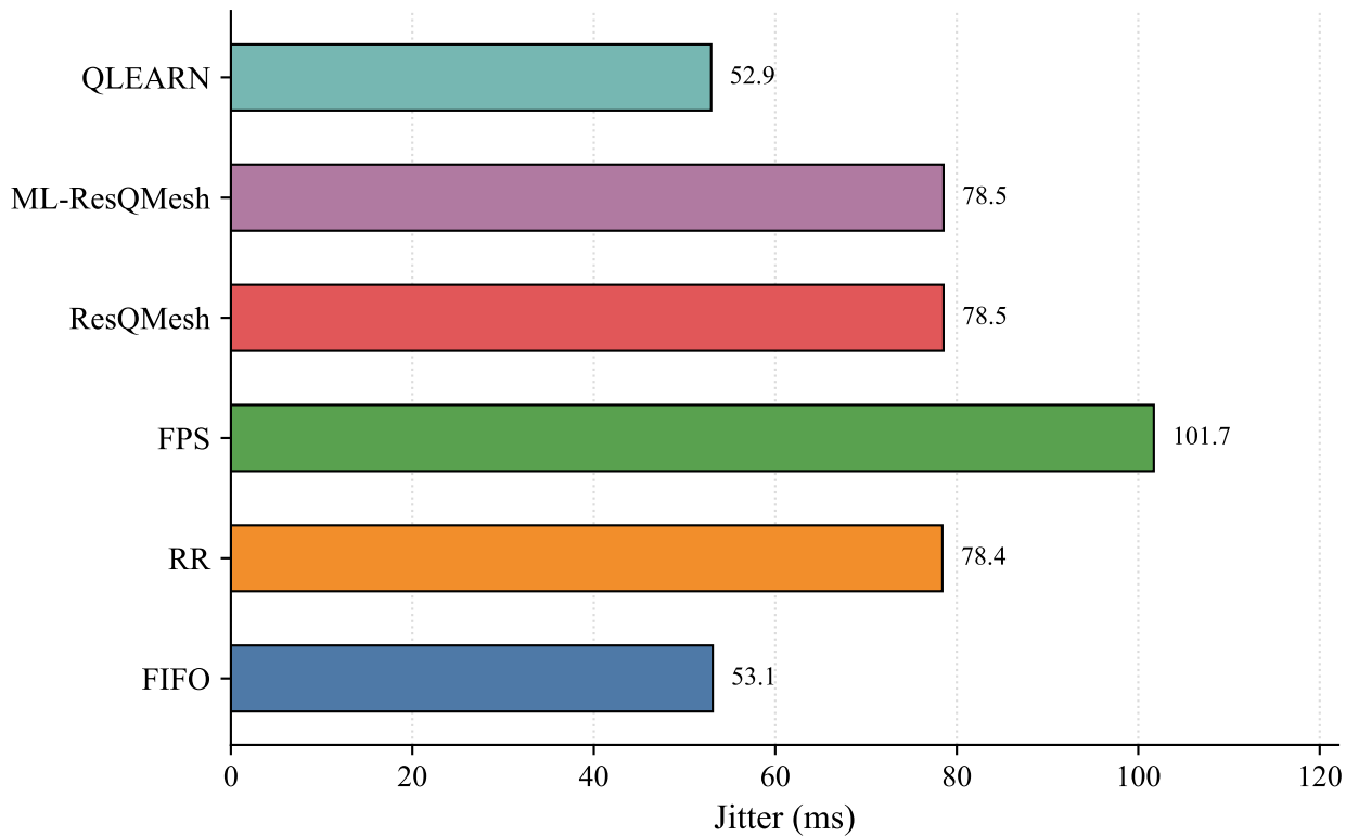
Jitter - Burst
