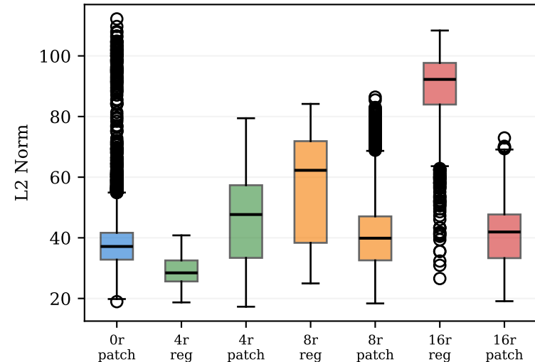
(d) Token Norm Distribution register vs patch tokens
