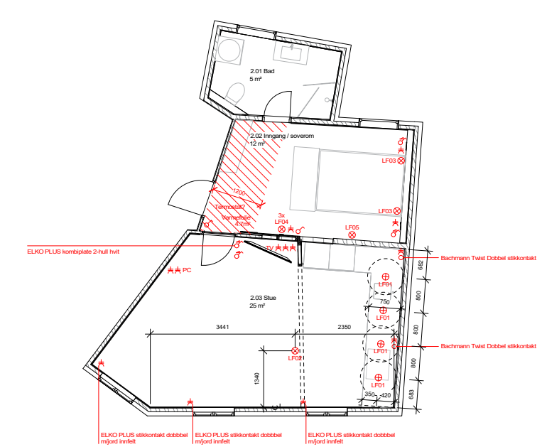
ELEKTROPLAN
