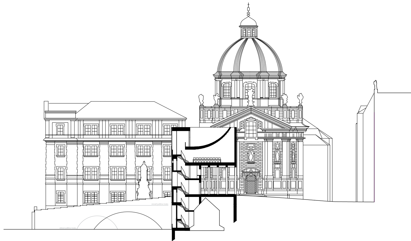
SNITT A-A
