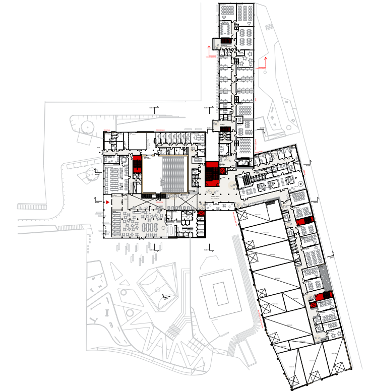
PLAN 02
