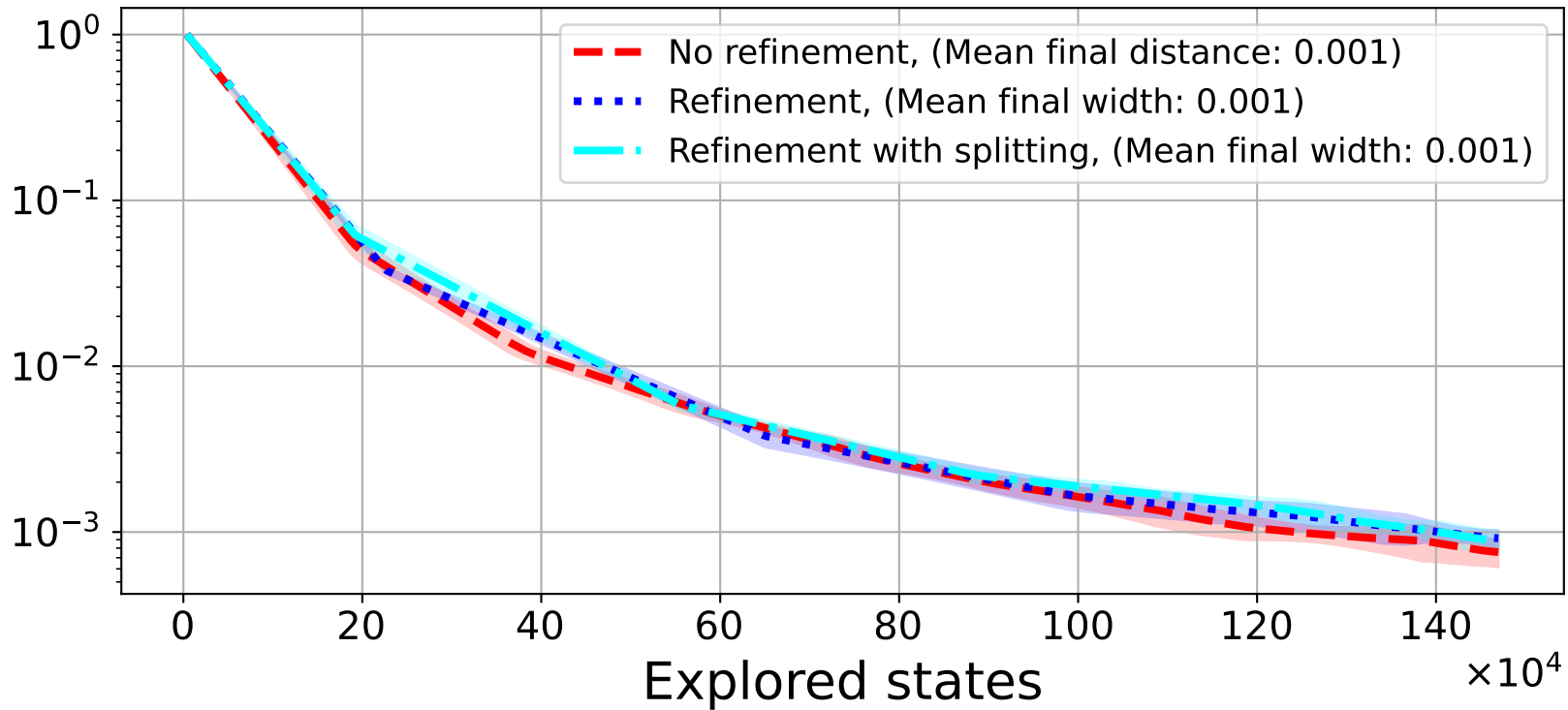
Interval Width
