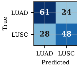
BoVW + SVM
