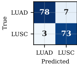
ABMIL (GigaPath)
