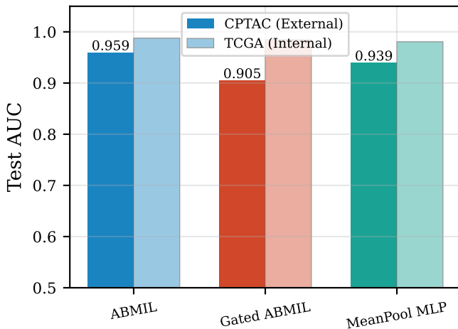
TCGA vs. CPTAC AUC
