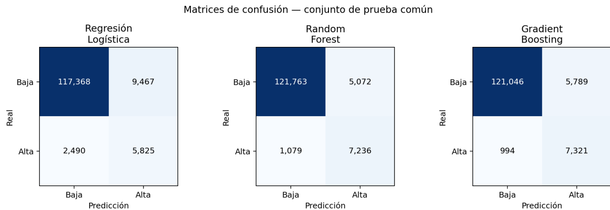
Figura 8: Matrices de confusión de los modelos ajustados sobre las mismas 135,150 observaciones de prueba.
