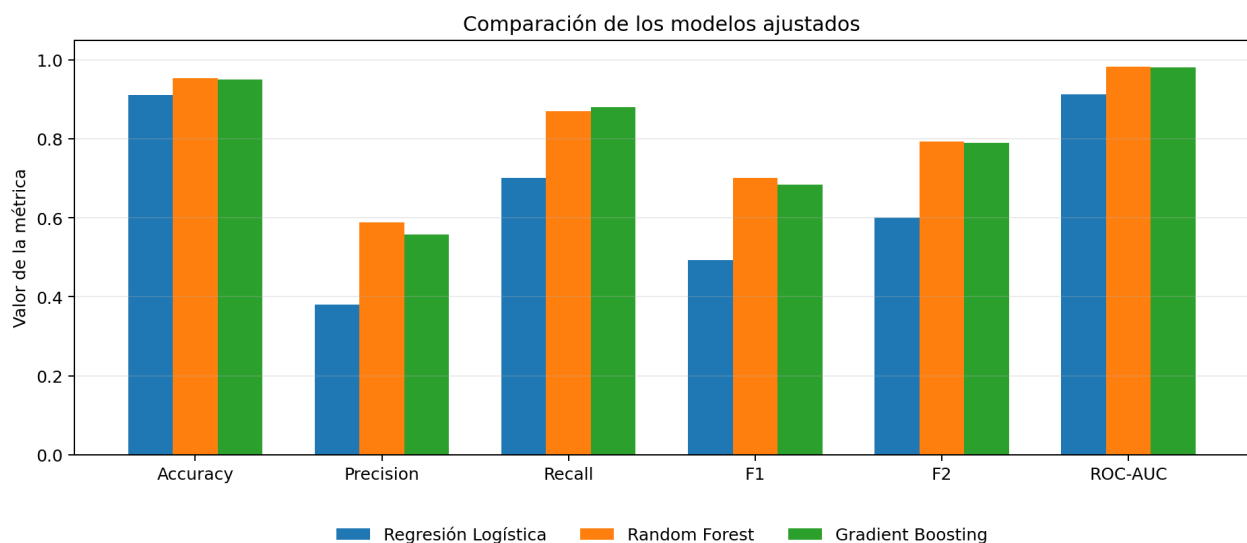
Figura 7: Comparación de las métricas finales. Random Forest y Gradient Boosting superan claramente a la Regresión Logística en recall , F1, F2 y ROC-AUC.
