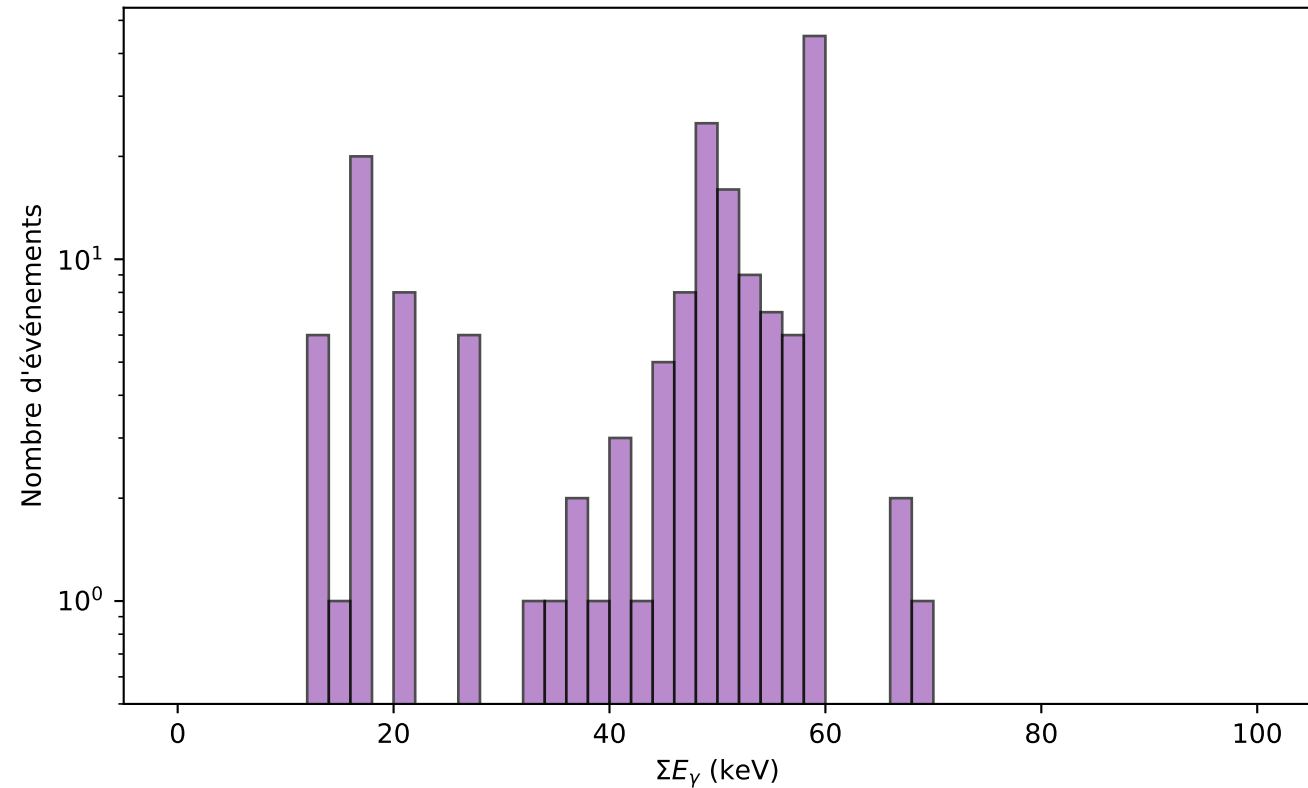
Énergie des photons rétrodiffusés
