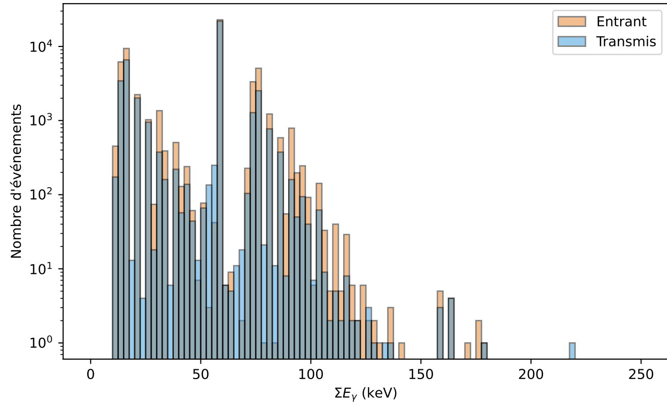
Comparaison \Sigma E_\gamma
