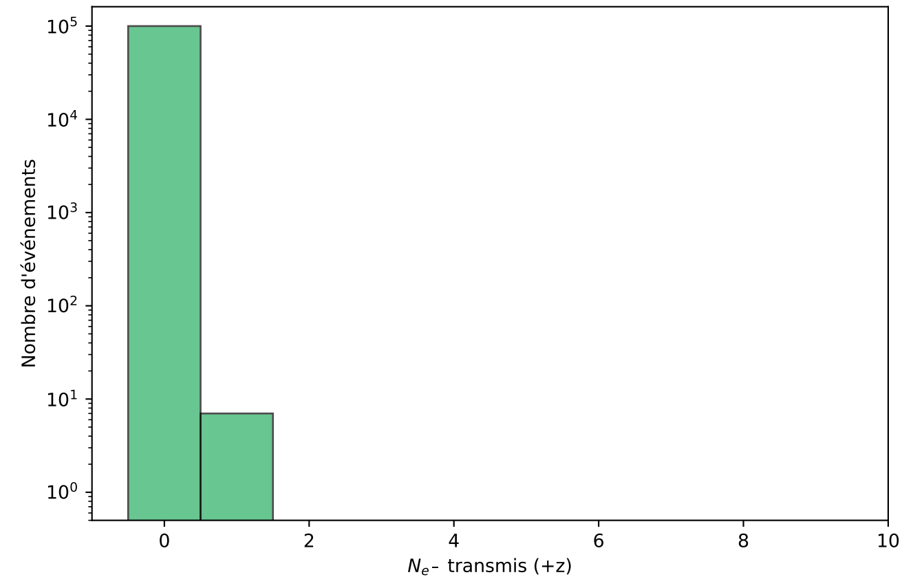
Électrons transmis - Nombre
