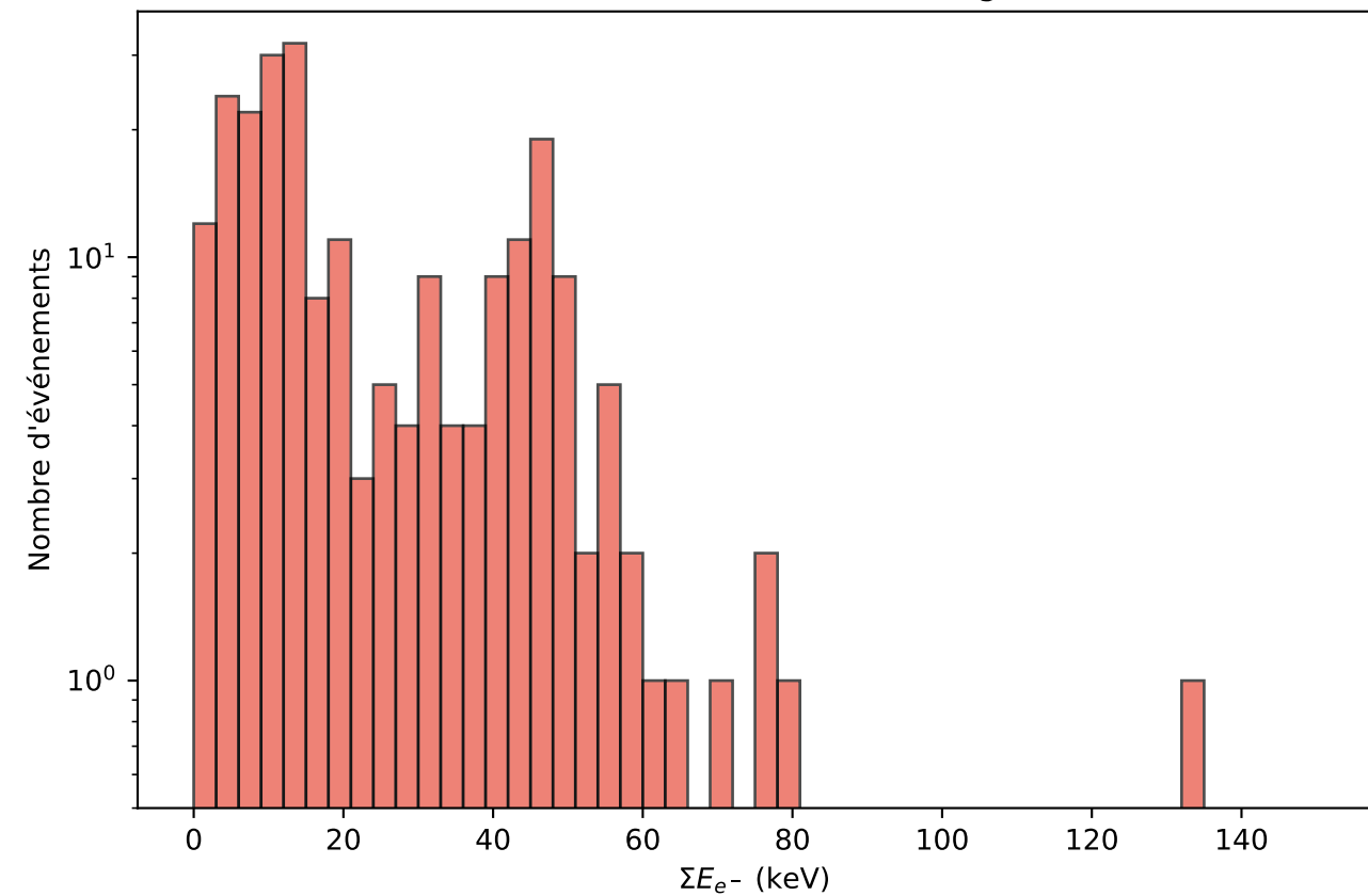
Électrons rétrodiffusés - Énergie
