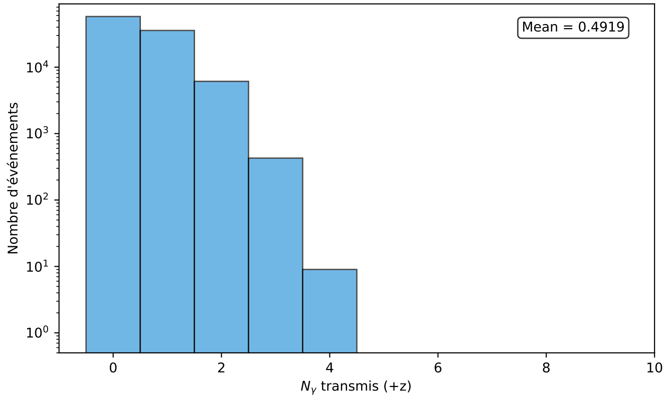
Nombre de photons transmis
