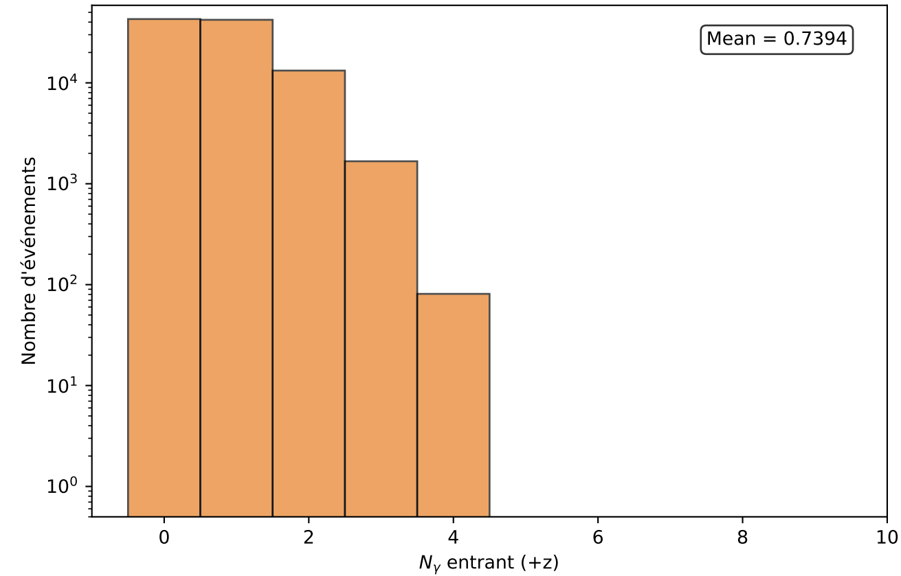
Nombre de photons entrant
