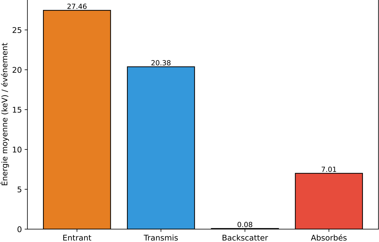
Bilan énergie photons
