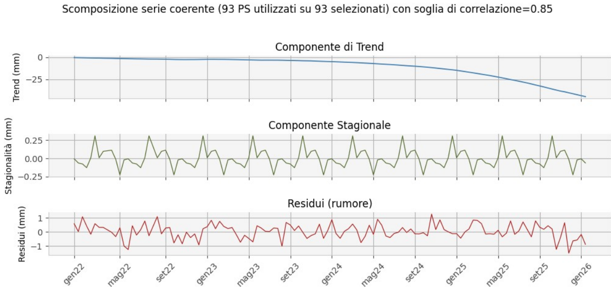
Fig. 6 — Scomposizione STL della serie media: dall'alto verso il basso, componente di trend T(t) , componente stagionale S(t) e residuo R(t) . L'entità della componente stagionale rispetto al trend indica il peso delle oscillazioni annuali sul segnale di deformazione.
