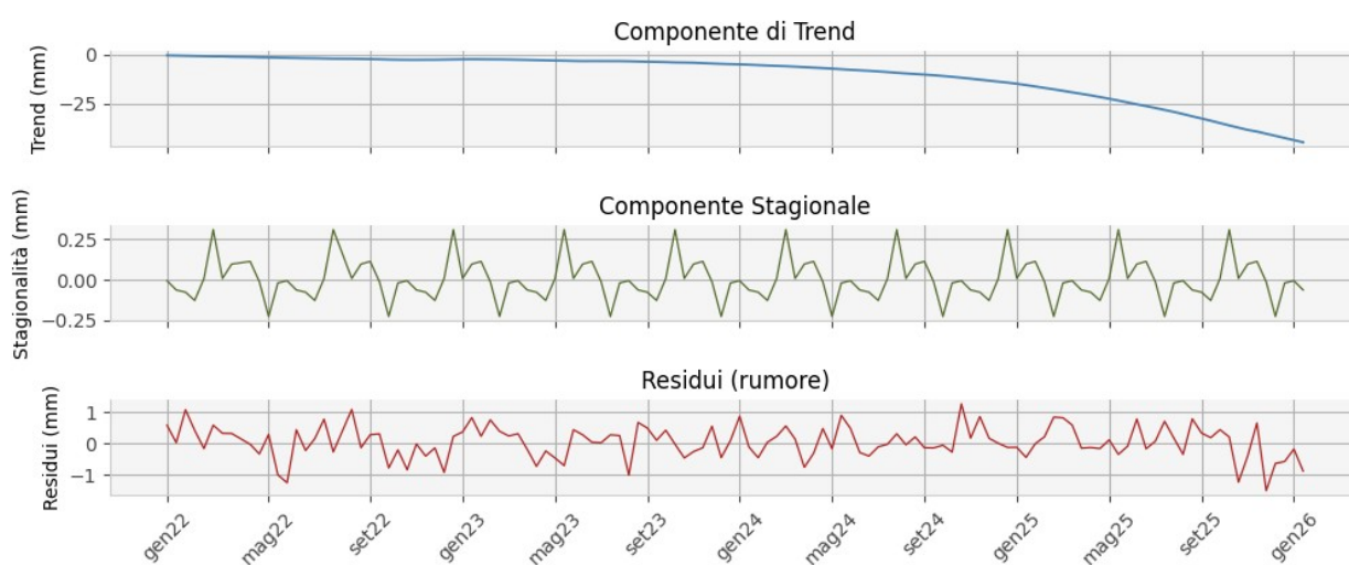
Fig. 6 — Scomposizione STL della serie media: dall'alto verso il basso, componente di trend T(t) , componente stagionale S(t) e residuo R(t) . L'entità della componente stagionale rispetto al trend indica il peso delle oscillazioni annuali sul segnale di deformazione.
