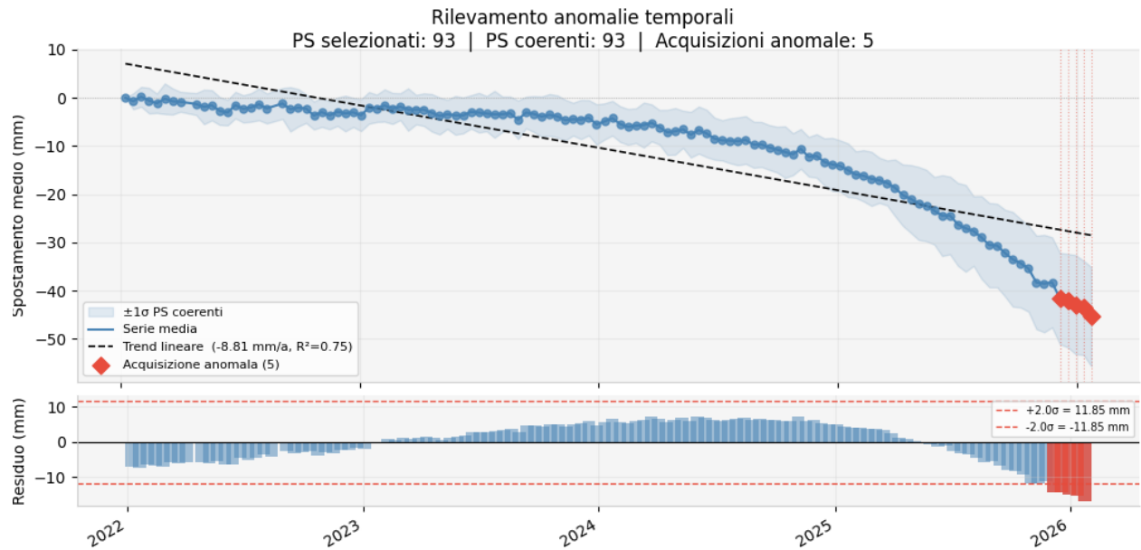
Fig. 8 — Rilevamento anomalie temporali: serie media con acquisizioni anomale (rombi rossi) e linee verticali tratteggiate rosse. Il grafico inferiore mostra i residui con le soglie di allerta. Il tooltip interattivo riporta data e spostamento con tag ANOMALIA per le acquisizioni fuori soglia.
