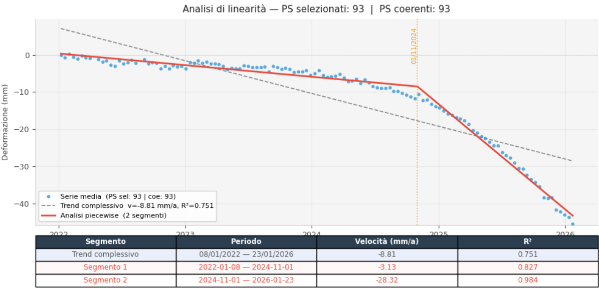
Fig. 7 — Analisi piecewise: serie media (punti blu) con trend complessivo (grigio tratteggiato) e modello lineare a tratti (rosso). I breakpoint sono indicati da linee verticali arancioni con la data corrispondente. La tabella riepilogativa in basso riporta periodo, velocità e R^2 per ogni segmento.
