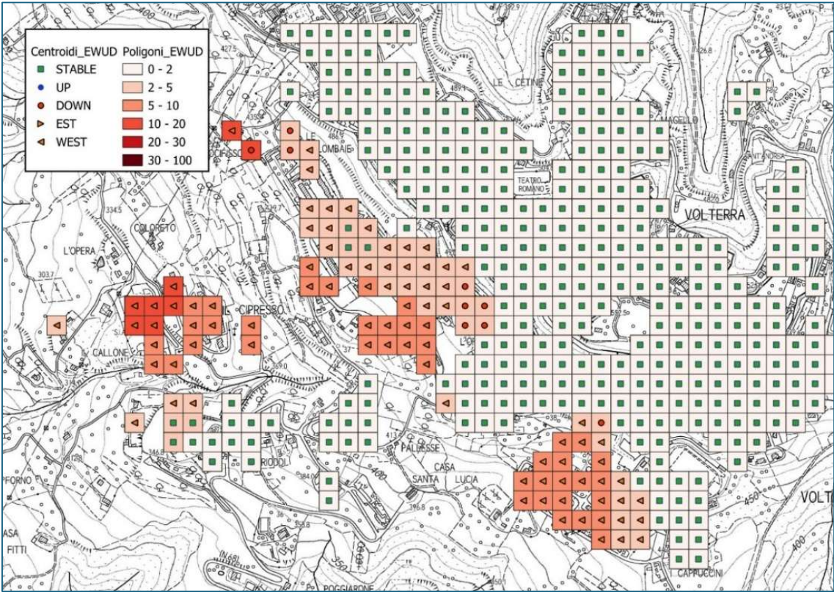
Fig. 2 — Layer Centroid_EWUD e Polygon_EWUD su mappa QGIS: i centroidi indicano la direzione prevalente del movimento nel piano EWUD e i poligoni sono colorati in scala cromatica in funzione della loro velocità nel piano EWUD espressa in mm/anno.
