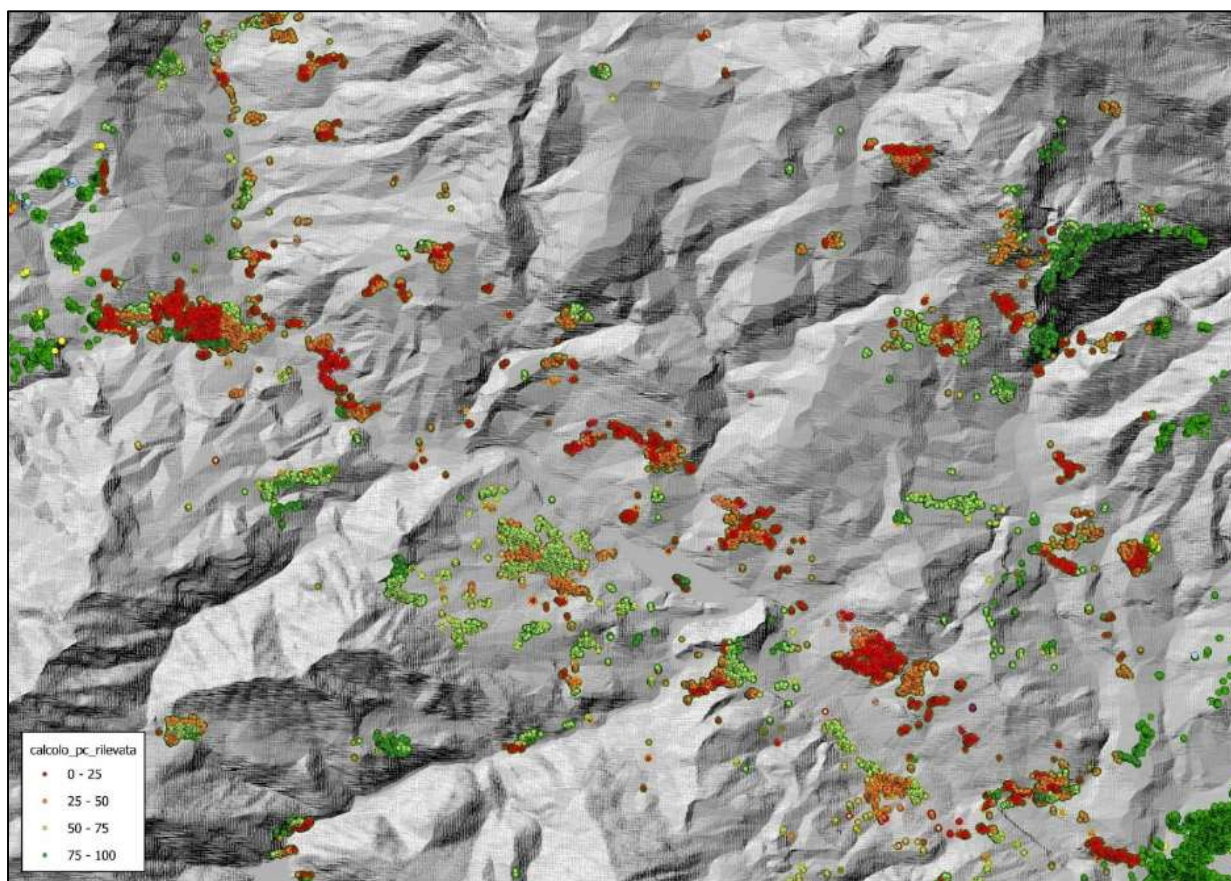
Fig. 3 — Mappa della percentuale di movimento rilevato da satellite ( pc_mov ) su layer PS ascendente: scala cromatica da rosso (bassa visibilità, movimento quasi perpendicolare alla LOS) a verde (alta visibilità, movimento quasi parallelo alla LOS). Sullo sfondo il DEM in hillshading.
