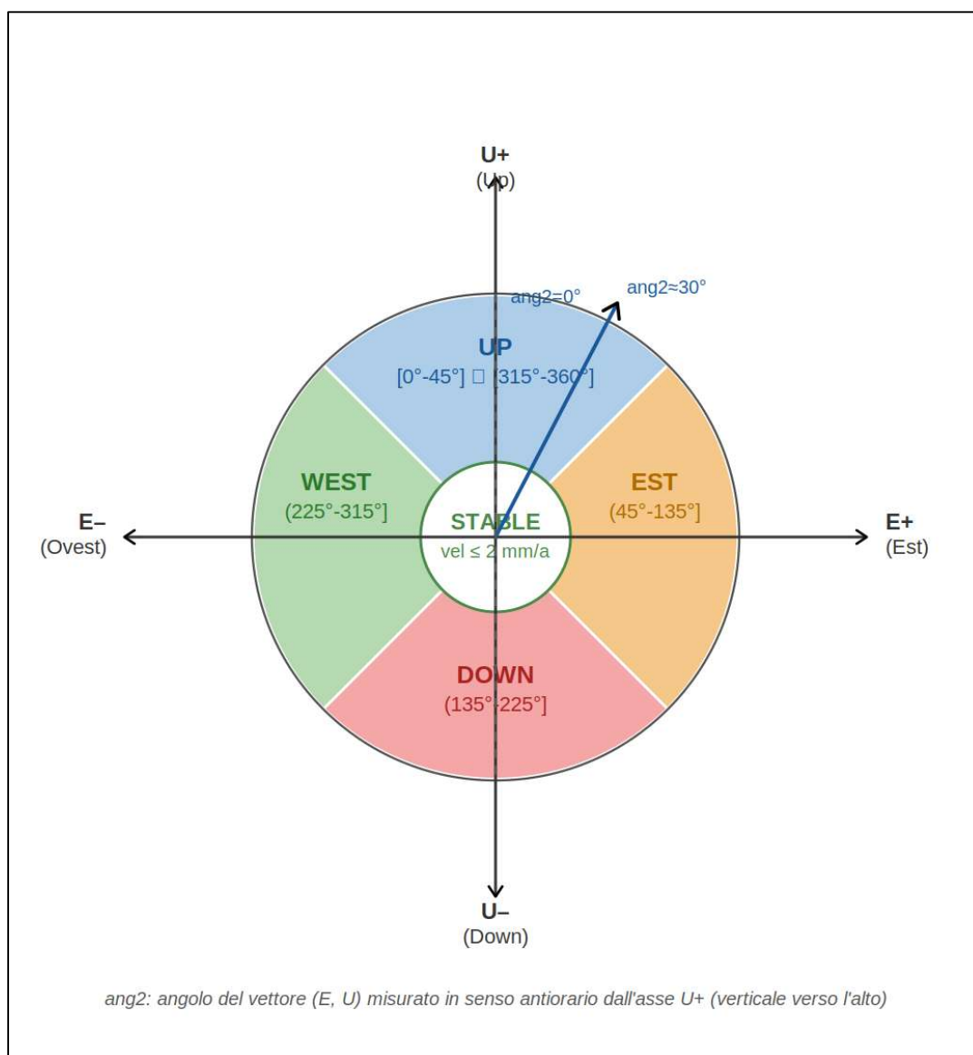
Fig. 1 — Schema della classificazione vprev in funzione dell'angolo ang2 del vettore velocità nel piano EW-UD. L'angolo ang2 è misurato in senso antiorario dall'asse U+ (verticale verso l'alto); la zona STABLE corrisponde a velocità vel \leq 2 mm/anno indipendentemente dalla direzione.
