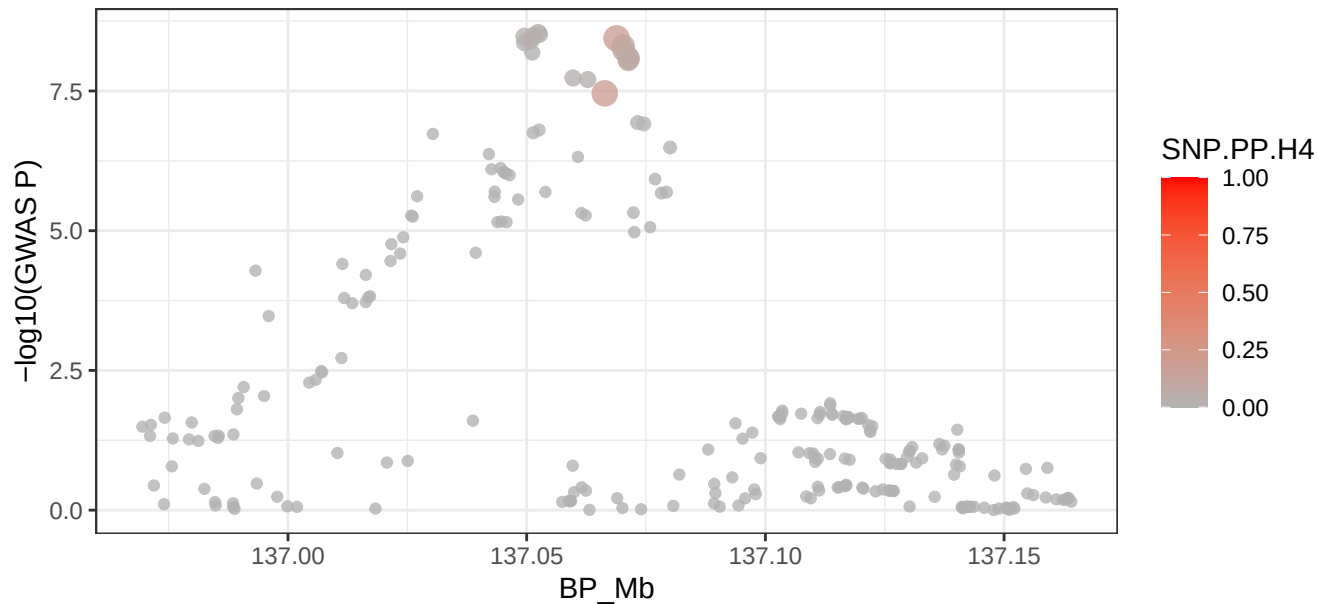
7_137067938 - edQTL
