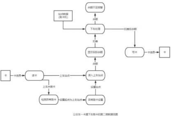
公交车一卡通下车刷卡的第二层数据流图
