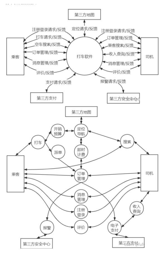
打车软件数据流图
