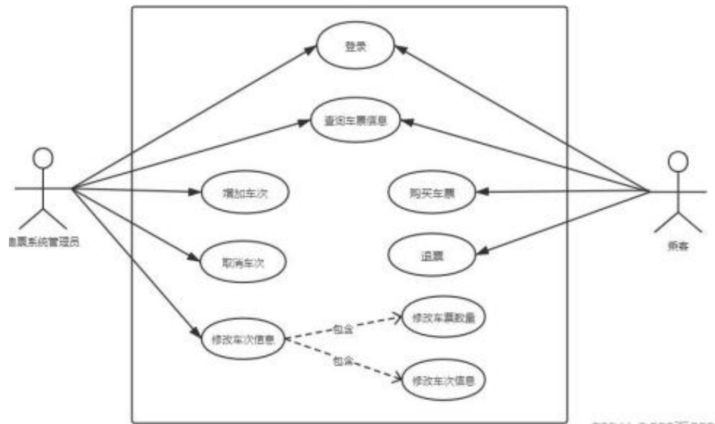
火车售票系统用例图
