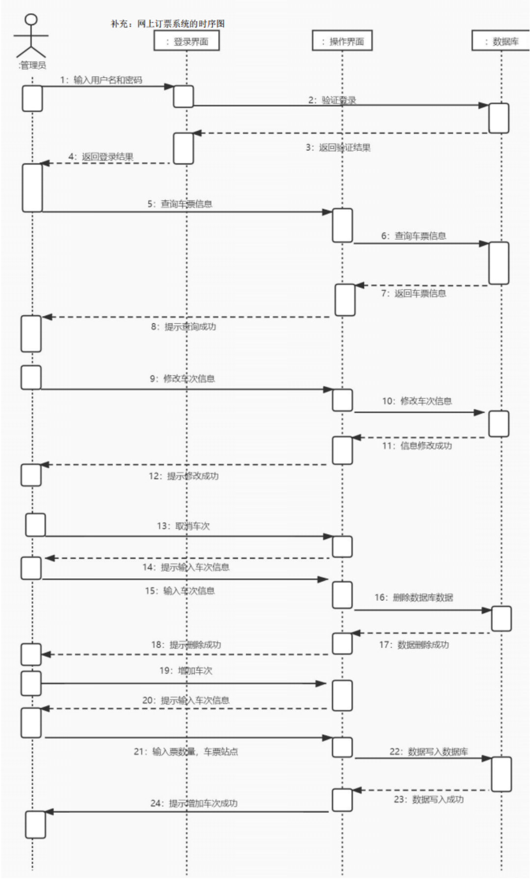
补充：网上订票系统时序图
