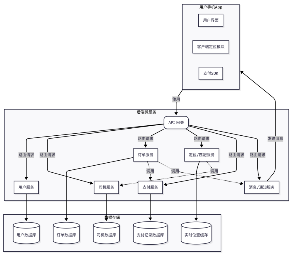
打车软件数据流图
