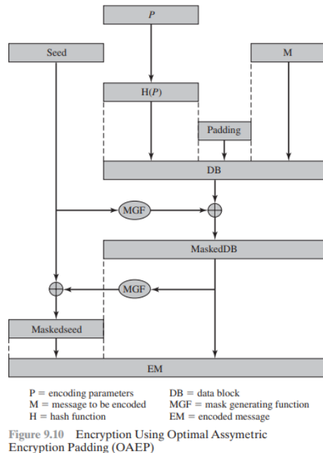
Figure 2.3: Sơ đồ khối quá trình nhào nặn dữ liệu của chuẩn OAEP (Nguồn: Figure 9.10)
