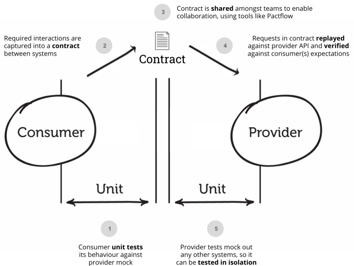
Schema de l'organisation des tests avec pact
