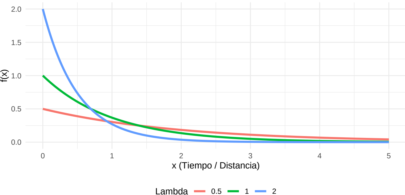
Figura 28. Función de densidad Exponencial Comparación para distintos valores de la tasa (.)
