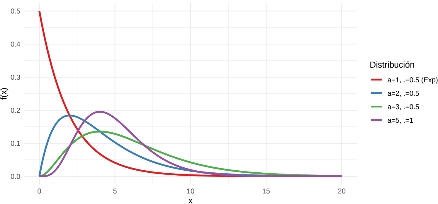
Distribución Gamma — distintos parámetros
