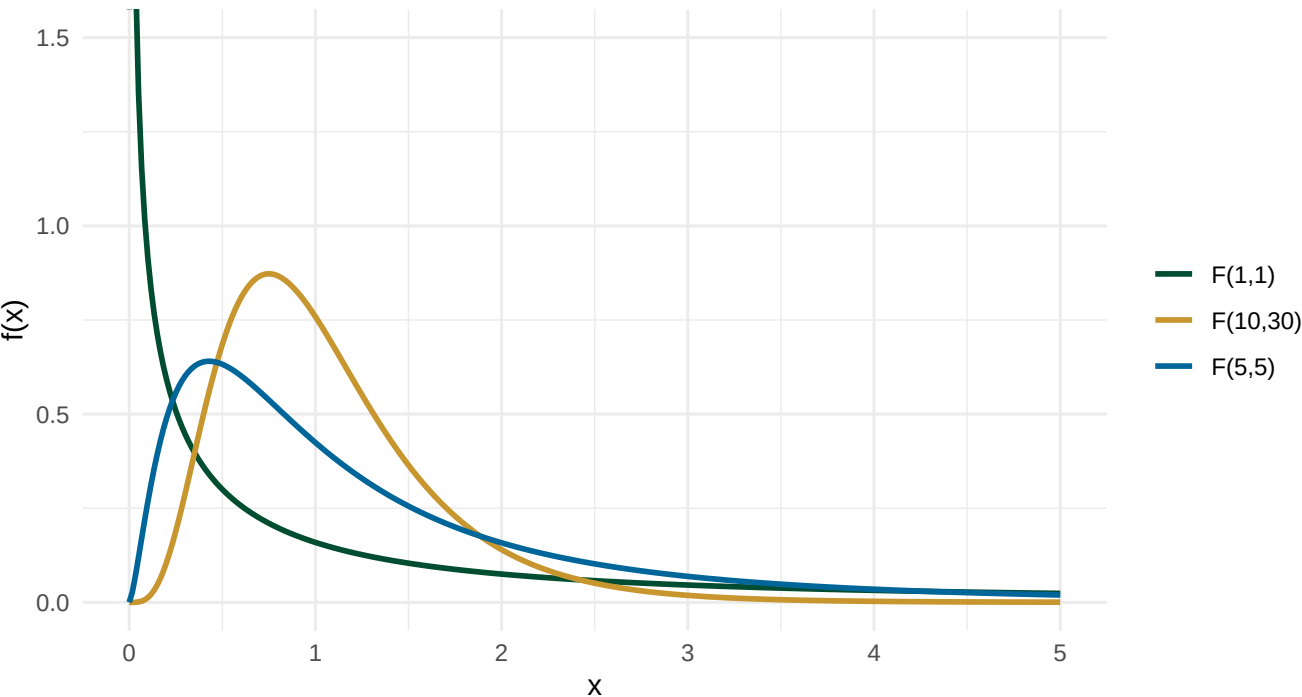
Distribución F para distintos grados de libertad
