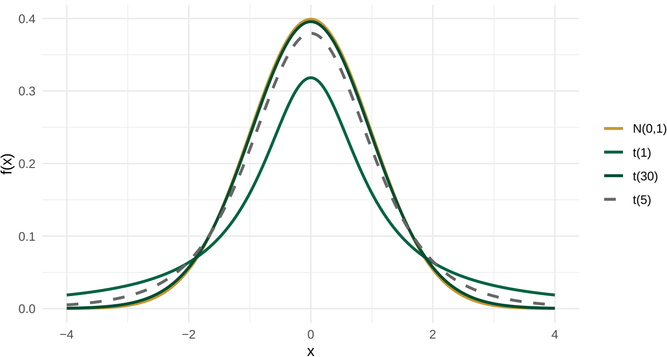
Distribución t de Student vs. Normal estándar
