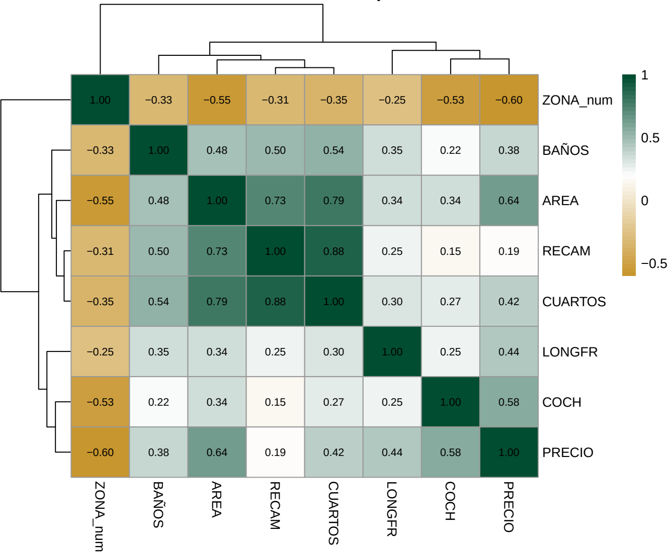
Matriz de correlación de Spearman
