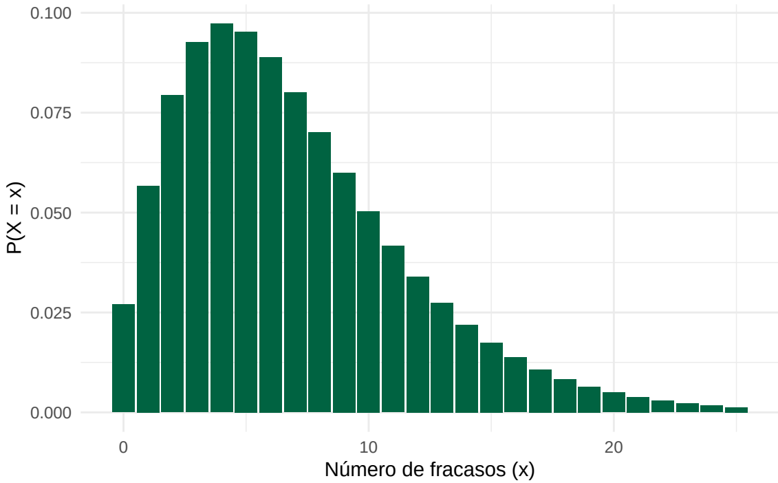
Binomial Negativa ( k = 3 éxitos, p = 0.3 )
