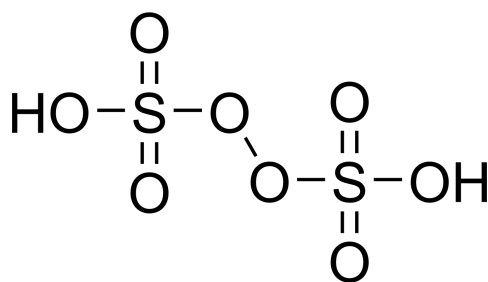
kyselina peroxodisírová
