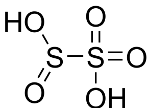
kyselina disiřičitá
