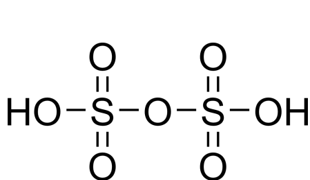
kyselina disírová
