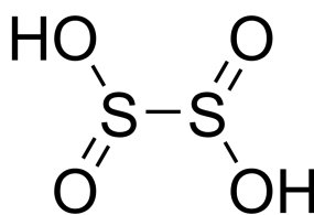
kyselina dithioničitá
