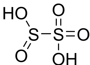
kyselina disiřičitá
