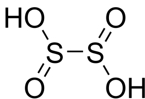
kyselina dithioničitá
