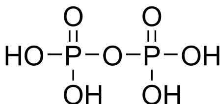
kyselina difosforečná
