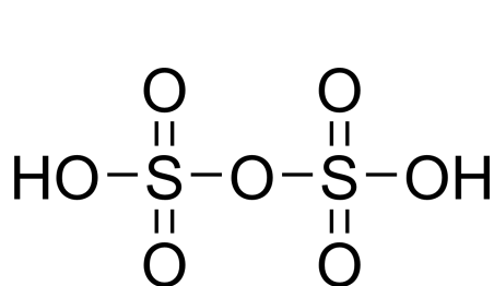
kyselina disírová
