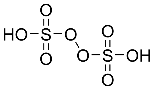
kyselina peroxodisírová
