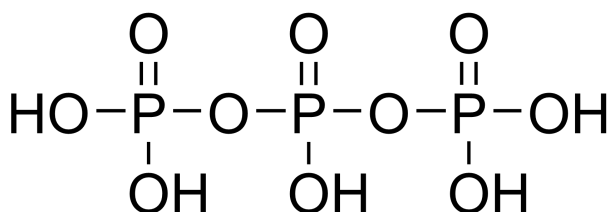
kyselina katena -trifosforečná
