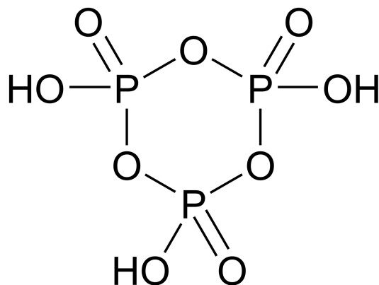
kyselina cyklo -trifosforečná
