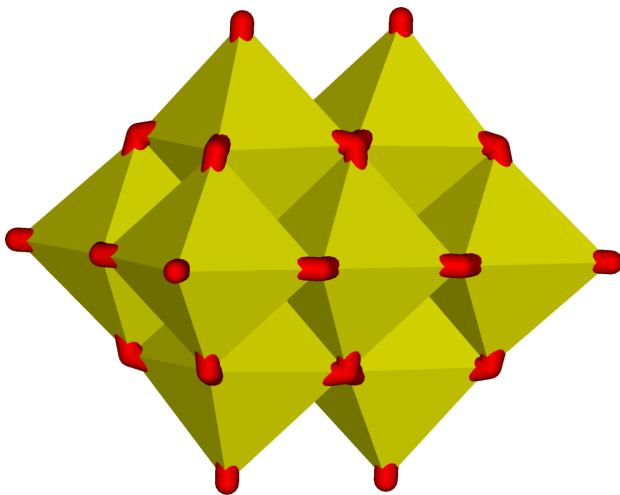
Struktura dekavanadičnanu [V_{10}O_{28}]^{6-} . 79
