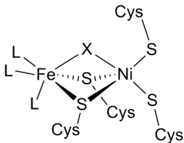
Aktivní místa NiFe hydrogenasy. 163
