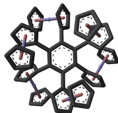
Hexaferrocenylbenzen. 142
