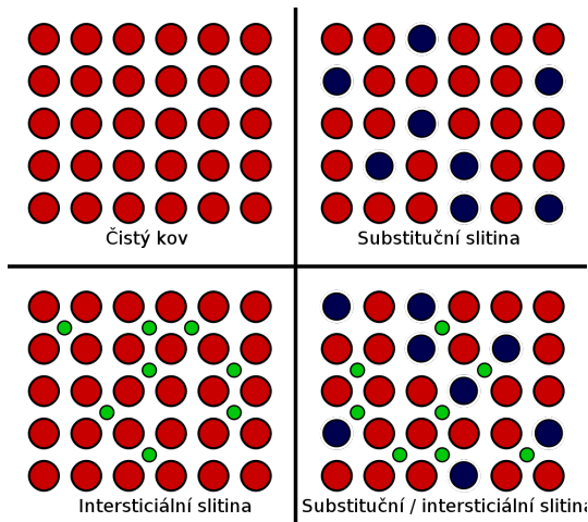
Typy slitin. 6
