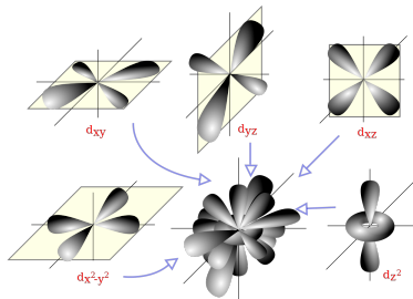
Tvary d-orbital . 39
