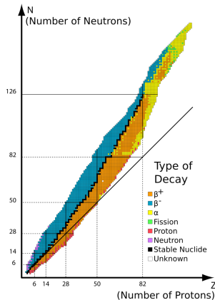
Typ rozpadu jádra v závislosti na protonovém čísle. 47
